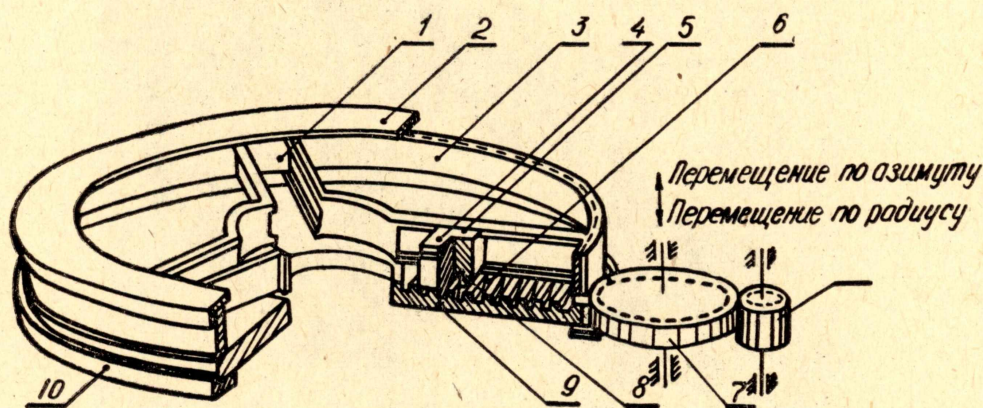
Рис. 1. Общий вид механизма
