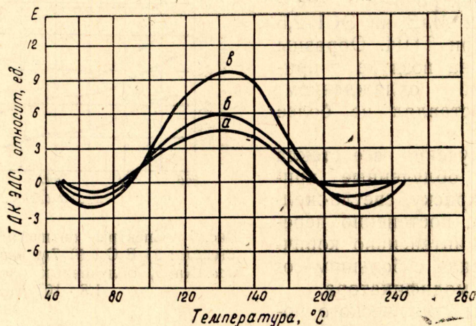
Рис. 3. Спектры ТДКэдс: а) B_2O_3 ; б) 3% вес. Na_2O ; в) 7% вес. Na_2O , облученных электронами дозой 1,8 \cdot 10^7 рад
