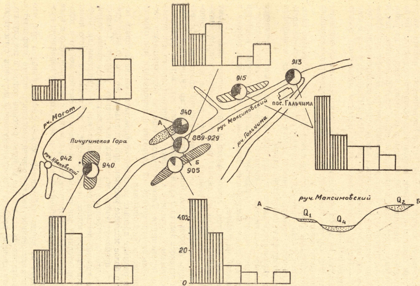
Рис. 2. Схема распределения золота с различной структурой в Максимовской группе россыпей.
