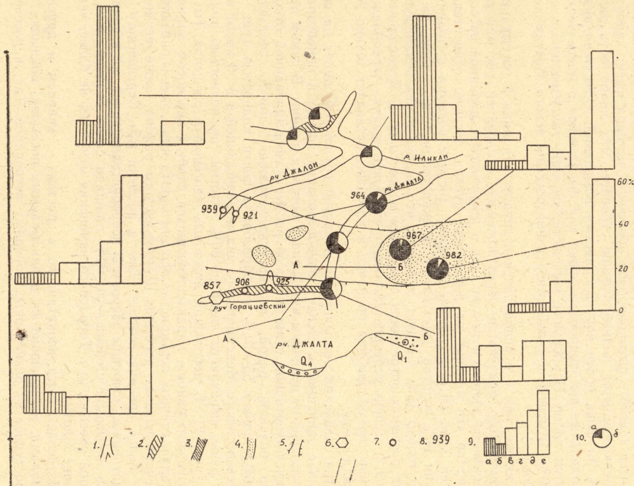
Рис. 1. Схема распределения золота различной структуры в Яснополянской группе россыпей
