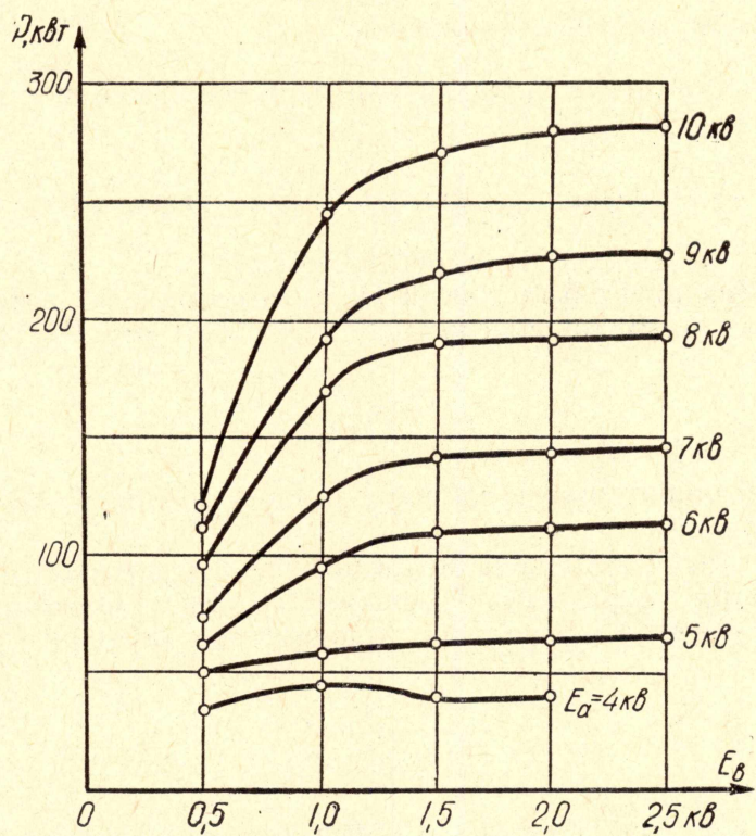
Рис. 4. Зависимость мощности генератора P_{\sim} = f(E_b) при E_a = \text{const} .
