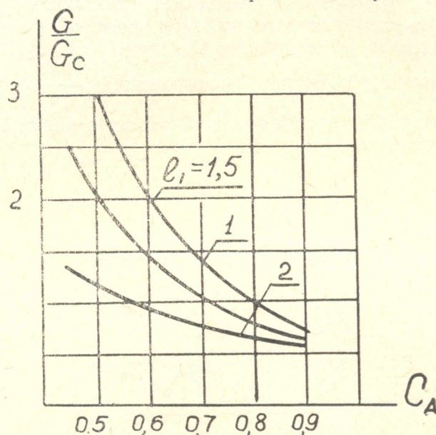
Рис. 3. Относительный вес совмещенной обмотки
