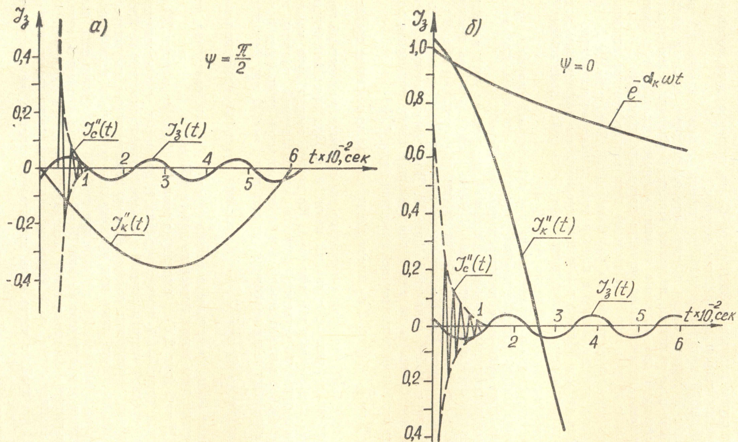
Рис. 2. Составляющие тока замыкания на землю для различных значений начальной фазы: а — при \Psi = \frac{\pi}{2} ; б — при \Psi = 0
