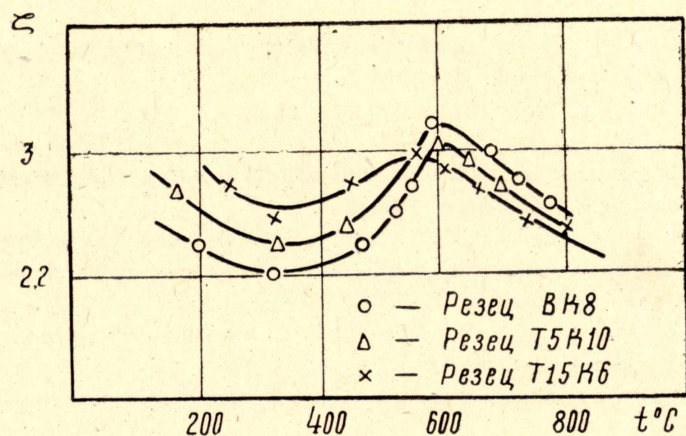
Рис. 1. Зависимость усадки стружки от средней температуры контакта при точении стали 08: \gamma=10^{\circ} ; t=2 мм; S=0,43 мм/об
