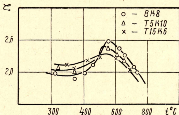
Рис. 2. Зависимость усадки стружки от средней температуры контакта при точении стали 45: \gamma=10^{\circ} ; t=2 мм; s=0,34 мм/об
