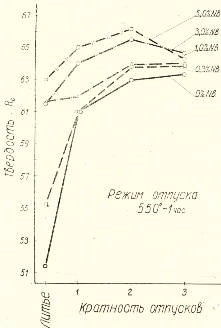
Рис. 2. Изменение твердости при отпуске литой быстрорежущей стали Р9 с содержанием углерода 1,4% и ниобия от 0 до 5%.
