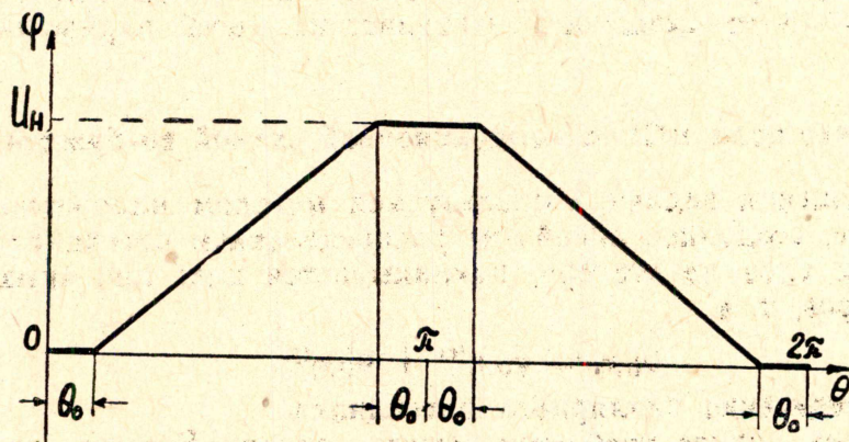
Рис. 2. Закон изменения потенциала статора
