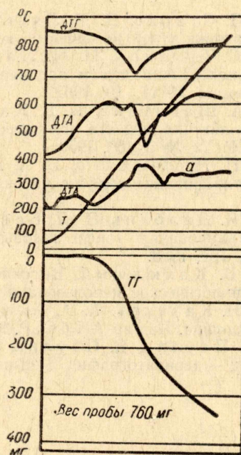
Рис. 4. Дериватограмма угля, бертинированного при 300°C. а) при загрузке образца в токе азота.
