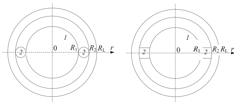
Рис. 2. Возможные представления поперечных сечений «снаряда» для системы с двумя каплями: 1 – высокотемпературные газы, 2 – капли
