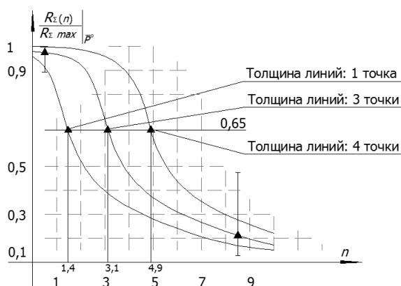
Рис. 3. Определение толщины контурной линии
