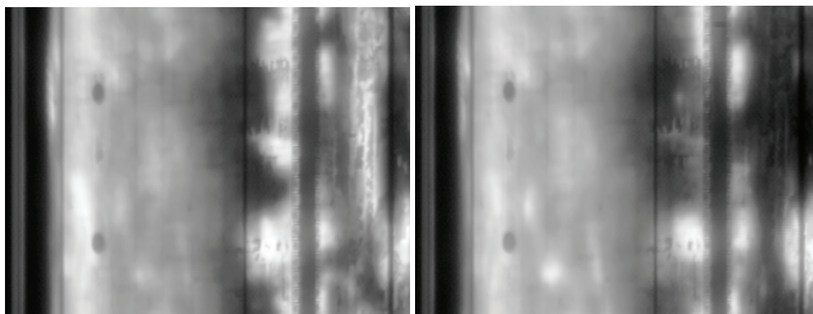
Рис. 1. Последовательность термограмм наружной поверхности печи в течение периода наблюдения (промежутки времени между термограммами 24 ч)
