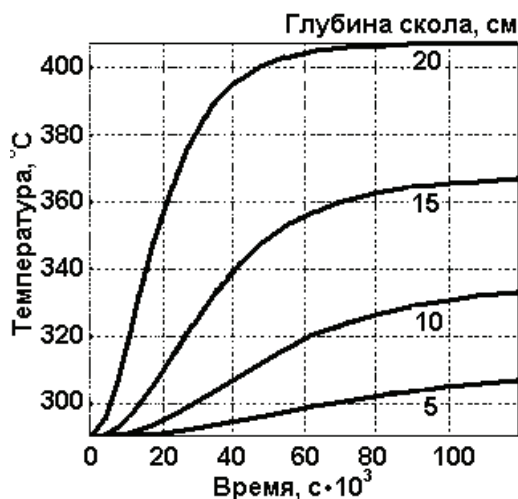
Рис. 3. Изменения температуры внешней поверхности, вызванные сколом обмазки различной глубины
