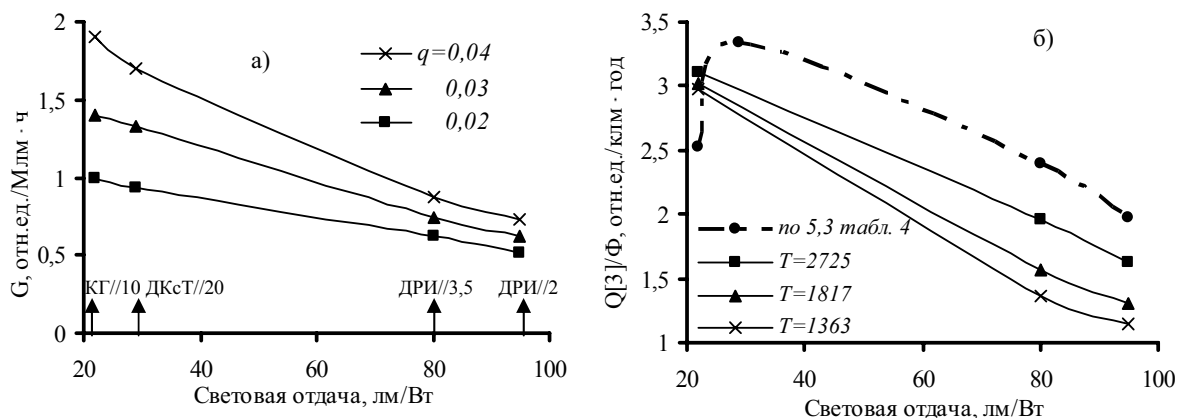
Рис. 1. Зависимость от световой отдачи: а) стоимости ЕСЭ при q=var ; б) приведенных затрат Q при T=var (штриховая линия по пункту 5.3 в табл. 4)
