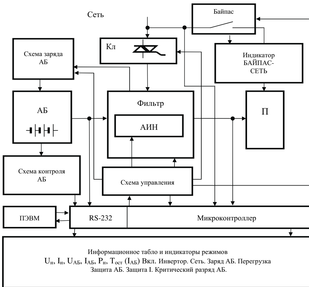
Рис. 4. Функциональная схема СБЭП (на примере ПОС-10000 АЛТЗ.211.211 ГНУ НИИ АЭМ)
