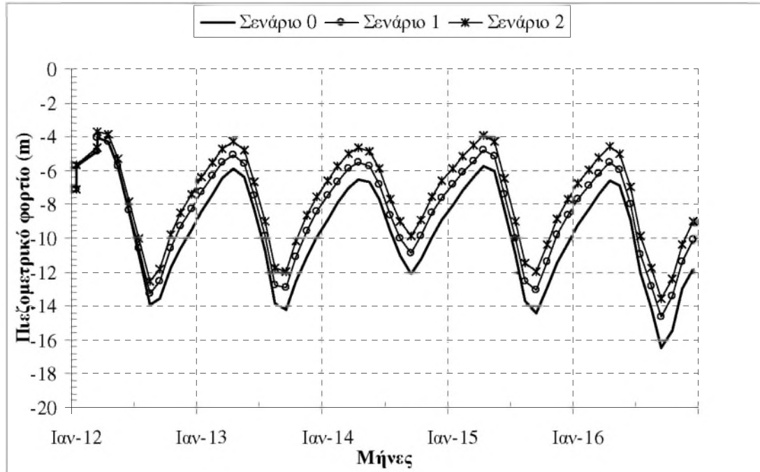
Σχήμα 2. Διακύμανση του πιεζομετρικού φορτίου των υπόγειων υδάτων του Ν. Ροδόπης (Σημείο 1)
