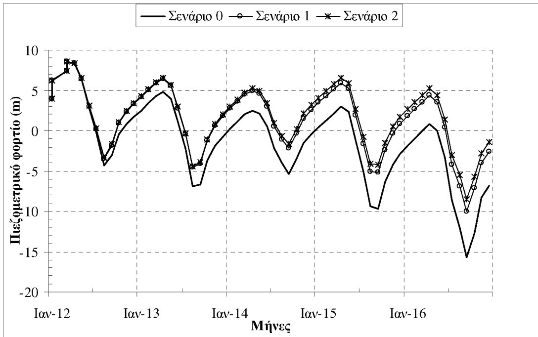
Σχήμα 7. Διακύμανση του πιεζομετρικού φορτίου των υπόγειων υδάτων του Ν. Ροδόπης (Σημείο 6)
