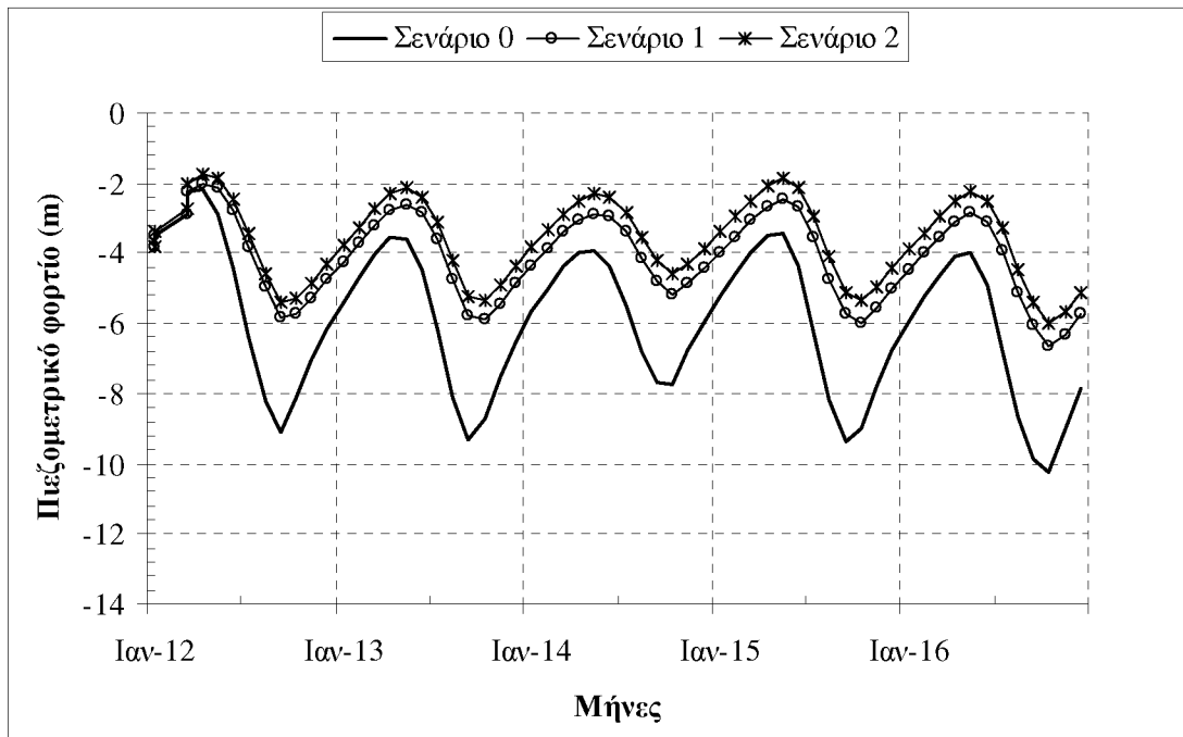
Σχήμα 8. Διακύμανση του πιεζομετρικού φορτίου των υπόγειων υδάτων του Ν. Ροδόπης (Σημείο 13)
