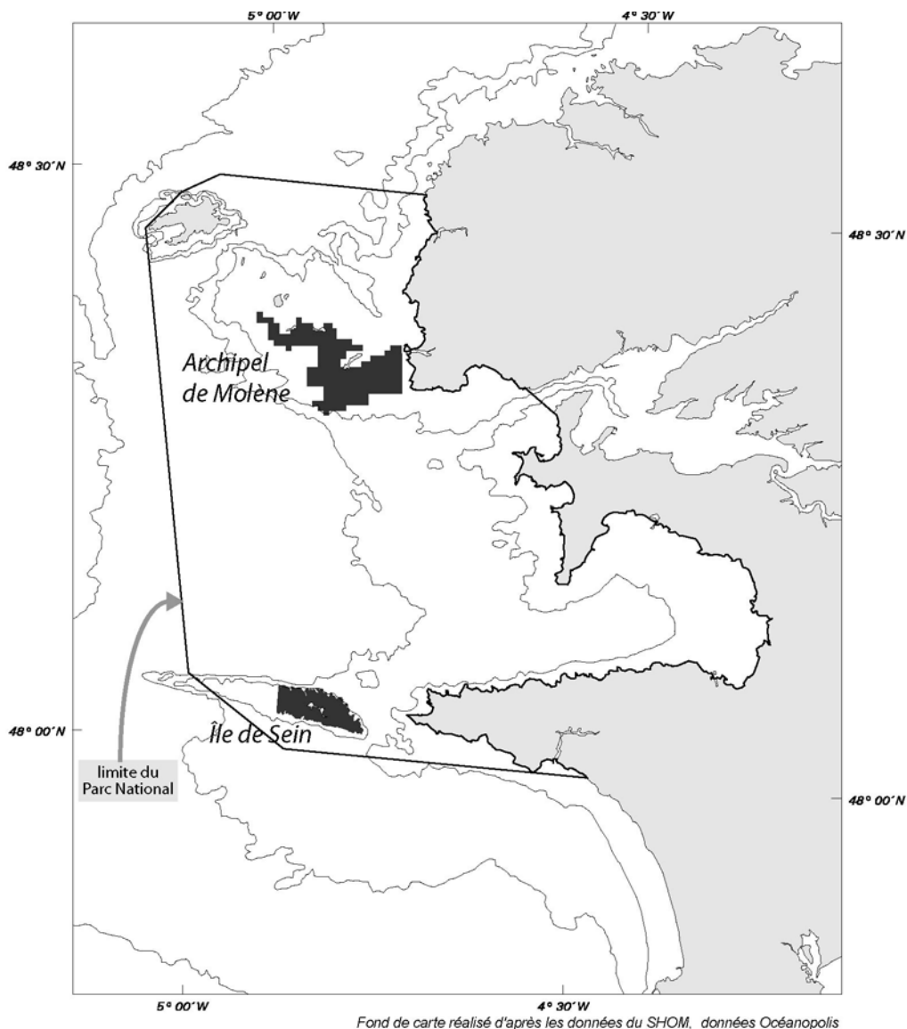
Illustration 60. La localisation des deux groupes de grands dauphins résidant en mer d'Iroise (d'après Liret et al. , 2003).
