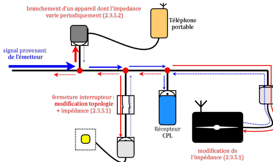
Figure 2.41 : Exemple de phénomènes aperiodiques.
