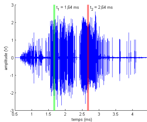
Figure 2.12: Bruit impulsif aperiodique - mesure de la DSP pour 2 instants.
