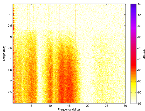
Figure 2.35 : Variation aperiodique du niveau de bruit stationnaire : Spectrogramme.
