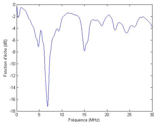
Figure 5.8 : Fonction d'écho du canal (paramètre S11).
