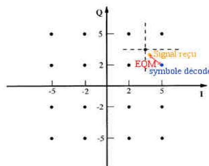
Figure 3.9 : Détection d'une impulsion par l'erreur quadratique moyenne.
