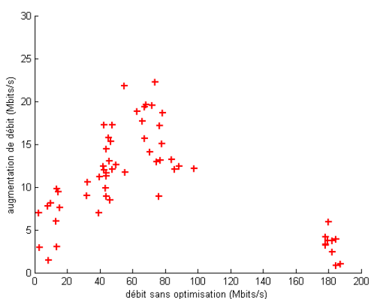
Figure 5.15 : Augmentation du débit (Mbits/s).
