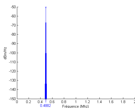
Figure VI.2 : Densité spectrale de puissance de la sinusoïde à 488,2 kHz.
