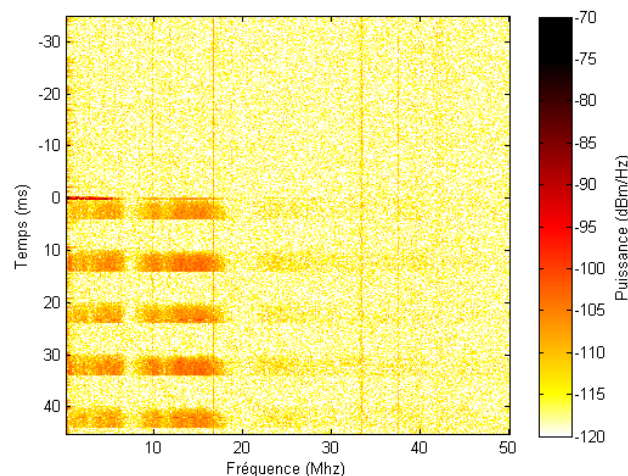
Figure 2.36 : Apparition de bruit impulsif périodique synchrone (spectrogramme).
