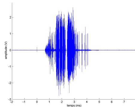
Figure 2.9 : Bruit impulsif a périodique.
