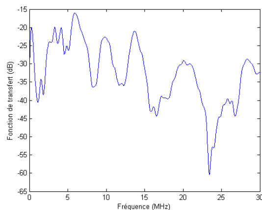
Figure 5.12 : Fonction de transfert des deux canaux.
