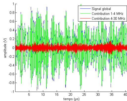
Figure 4.8 : Contribution des fréquences sur l'amplitude du spectre.
