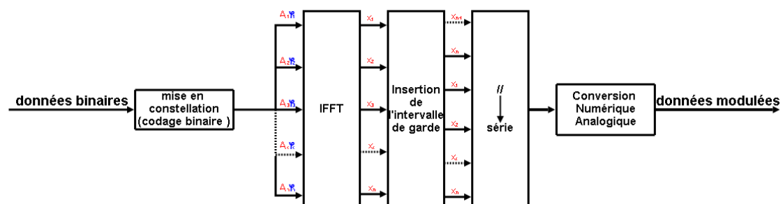
Figure 1.15 : Modulateur OFDM bande de base.
