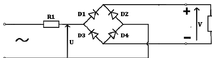
Figure VIII.1 : Pont de Graëtz.
