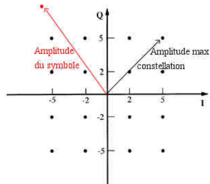
Figure 3.8 : Détection d'une impulsion par l'amplitude sur une porteuse.
