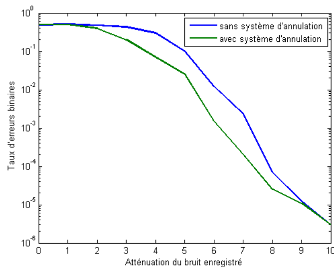
Figure 3.42 : Performances de l'algorithme d'annulation.
