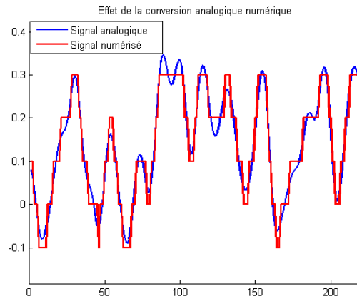
Figure III.1 : Effet de la conversion Analogique/Numérique sur le signal.
