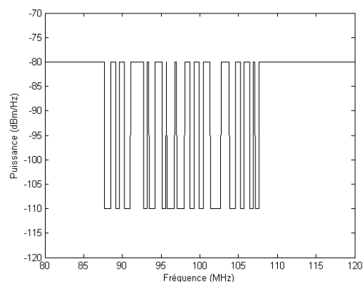
Figure 5.6 : Masque d'émission bande 80-120 MHz obtenu à partir de la base de données [65].
