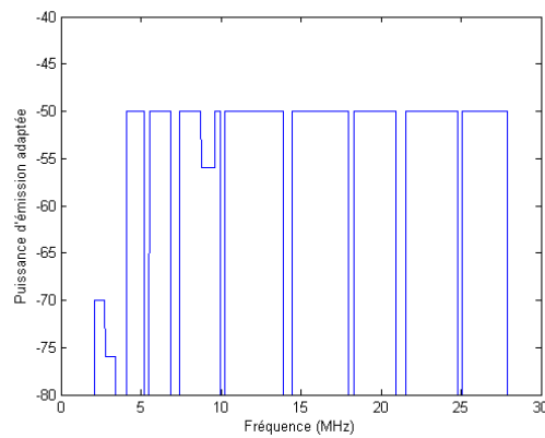
Figure 4.9 : Masque d'émission optimisé.
