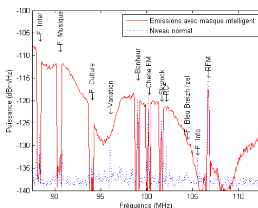
Figure 5.5 : Puissance reçue en présence de notches intelligentes.
