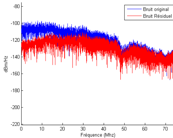
Figure 3.30: Comparaison du bruit original et du bruit résiduel après annulation.
