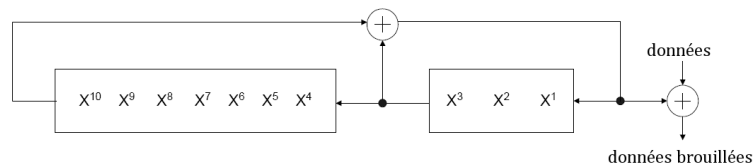
Figure 1.21 : Brouilleur de données.
