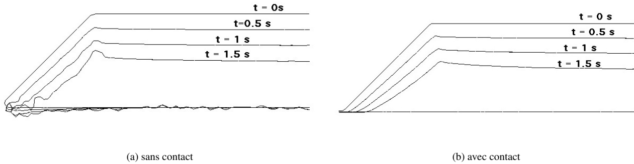
FIG. 8: Evolution de l'interface simulés en 2D
