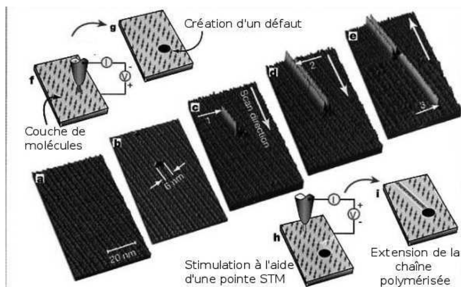
FIG. 1.18 – (a) couche monomoléculaire d'acide 10,12-nonacosadiynoïc, (b) création d'un défaut, (c) première chaîne polymérisée, initialisée au point indiqué par la flèche (1) en utilisant la pointe du STM, (d) seconde chaîne polymérisée, (e) troisième chaîne polymérisée.
