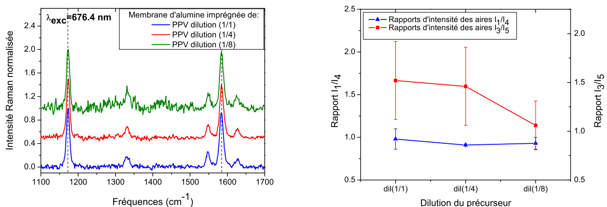
FIG. 4.23 – A gauche : spectres de diffusion Raman obtenus sur des tranches d'alumine imprégnées de PPV issu de dilution (1/1), (1/4 et (1/8) ; à droite : rapports d'intensité des aires de bandes Raman ; \lambda_{exc} = 676,4 \text{ nm} .
