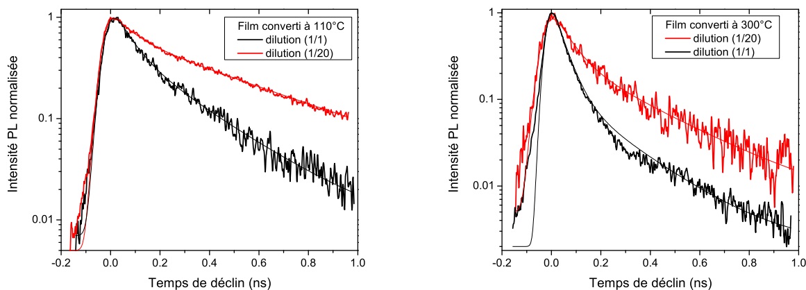
FIG. 3.13 – Déclins de PL de films de PPV issus d'une dilution du précurseur (1/1) et (1/20) convertis à 110°C (à gauche) et convertis à 300°C (à droite).
