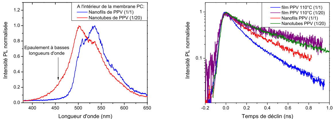
FIG. 4.13 – A gauche : spectres de PL de nanofils de PPV (issus de dilution (1/1) du précurseur) et de nanotubes de PPV (issus de dilution (1/20) du précurseur). A droite : Déclin de PL des nanofils et des nanotubes de PPV. Les nanofibres sont étudiées dans la membrane PC. Les déclin de film de PPV convertis à 110^\circ\text{C} issus de dilutions (1/1) et (1/20) sont également ajoutés pour comparaison ; \lambda_{exc}=267 nm.
