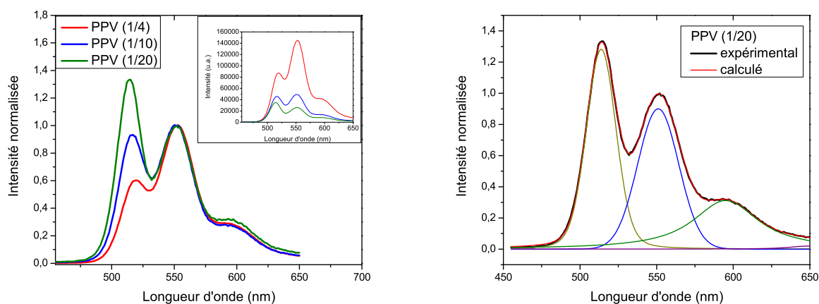
FIG. 3.6 – A gauche : spectres de photoluminescence normalisés de film PPV en fonction de la dilution (non normalisés dans l'encart), \lambda_{exc} = 440nm . A droite : Déconvolution du spectre de PL du film issu d'une dilution (1/20) du précurseur.
