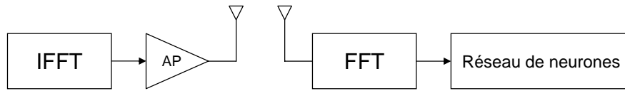
FIGURE 3.2 – Schéma simplifié de la méthode réduction des non linéarités par réseaux de neurones
