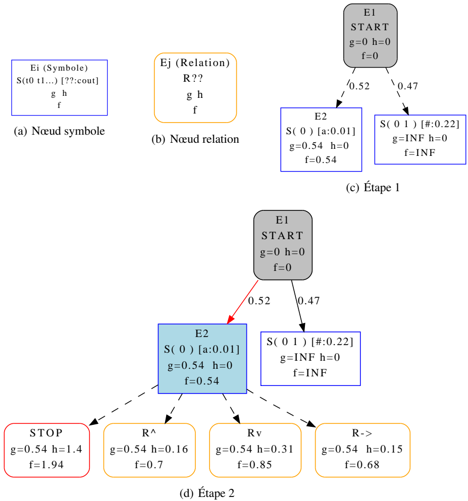
Figure 2. Les deux types de nœuds sont illustrés par (a) et (b). Les figures (c) et (d) présentent l'état du graphe aux étapes E1 et E2 du tableau 1. Les nœuds pleins sont les nœuds visités au cours de l'algorithme. Les arcs rouges symbolisent le meilleur chemin courant, et les arcs pointillés relient le nœud courant avec les nœuds créés à l'étape considérée.
