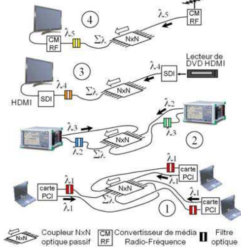
Fig. 1: Configuration du réseau réalisé
