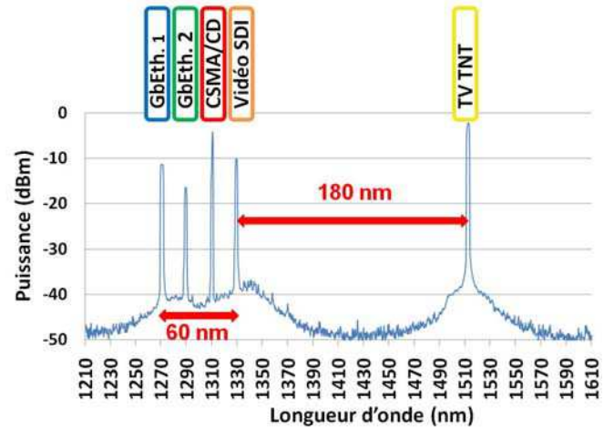
Fig. 2: Spectre des longueurs d'onde implémentées
