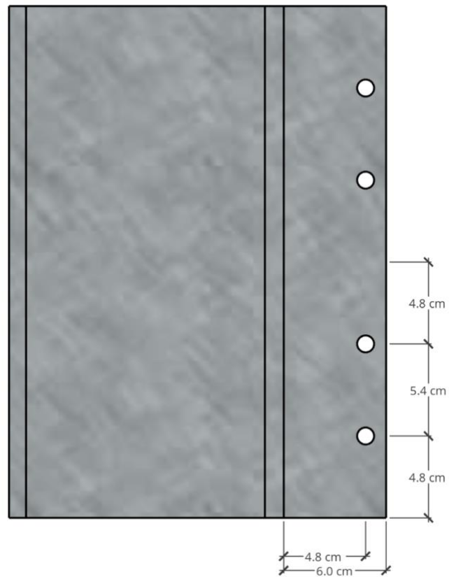
Figur 23 Mål for plassering av skruer sett ovenfra. Tegnet i Sketchup.
