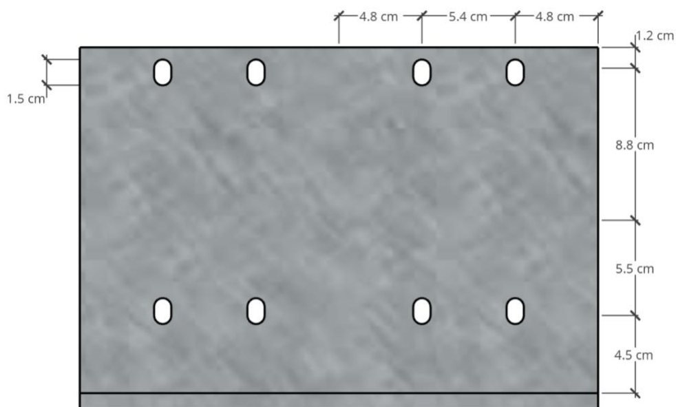
Figur 22 Mål for plassering av skru hull sett fra siden. Tegnet i Sketchup
