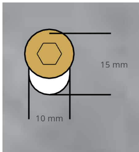
Figur 24 Dimensjoner av avlange skruer i vertikal retning. Tegnet i Sketchup
