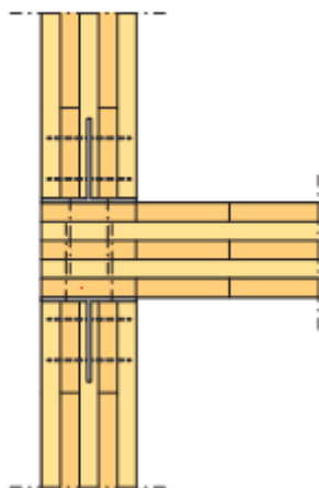
Figur 6 Skjulte metallplater, [2]
