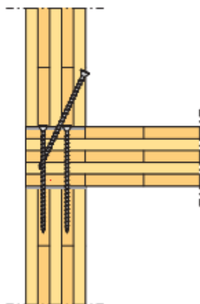
Figur 4 Selvborende skruer [2]
