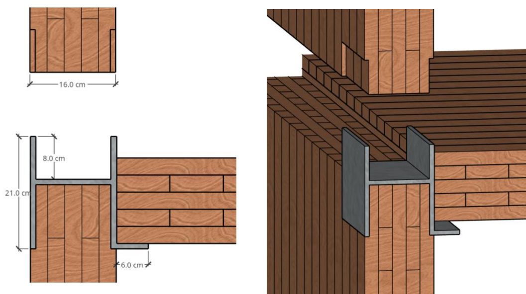
Figur 12 Endelig design for yttervegg med mål.
