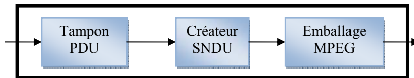
Figure 2.4: Structure de l'encapsulateur IP
