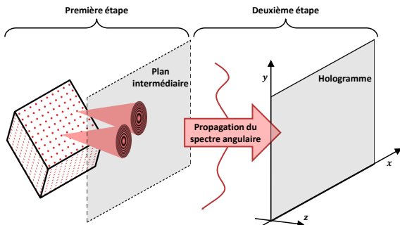
FIGURE 7 – Réduction de la complexité du calcul de l’onde objet par la méthode du plan intermédiaire : l’onde lumineuse issue de chacun des points de la scène est calculée dans le plan intermédiaire, puis propagée dans le plan de l’hologramme par la formule du spectre angulaire.
