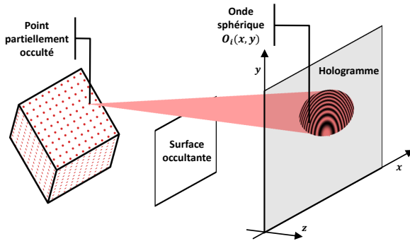
FIGURE 5 – Prise en compte des occultations lors du calcul de l’onde objet par analyse géométrique de la scène : la région de contribution du point lumineux dans le plan de l’hologramme est réduite à cause de la surface occultante.
