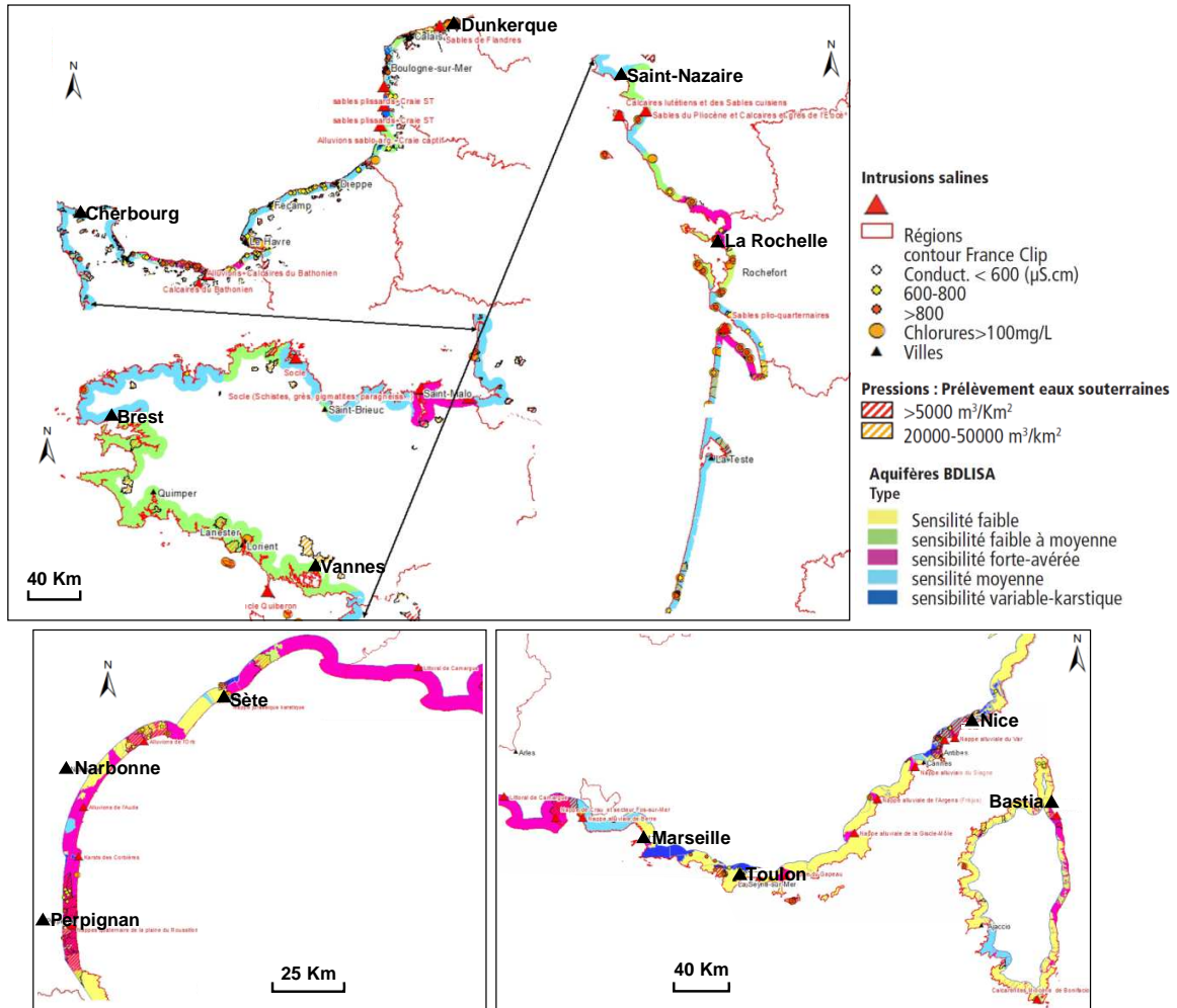
Figure IV.9 Carte de vulnérabilité des aquifères côtiers en France Métropolitaine à la remontée du niveau marin de +2 m et pression par prélèvements. Source : Dörfliker et al. (2011).
