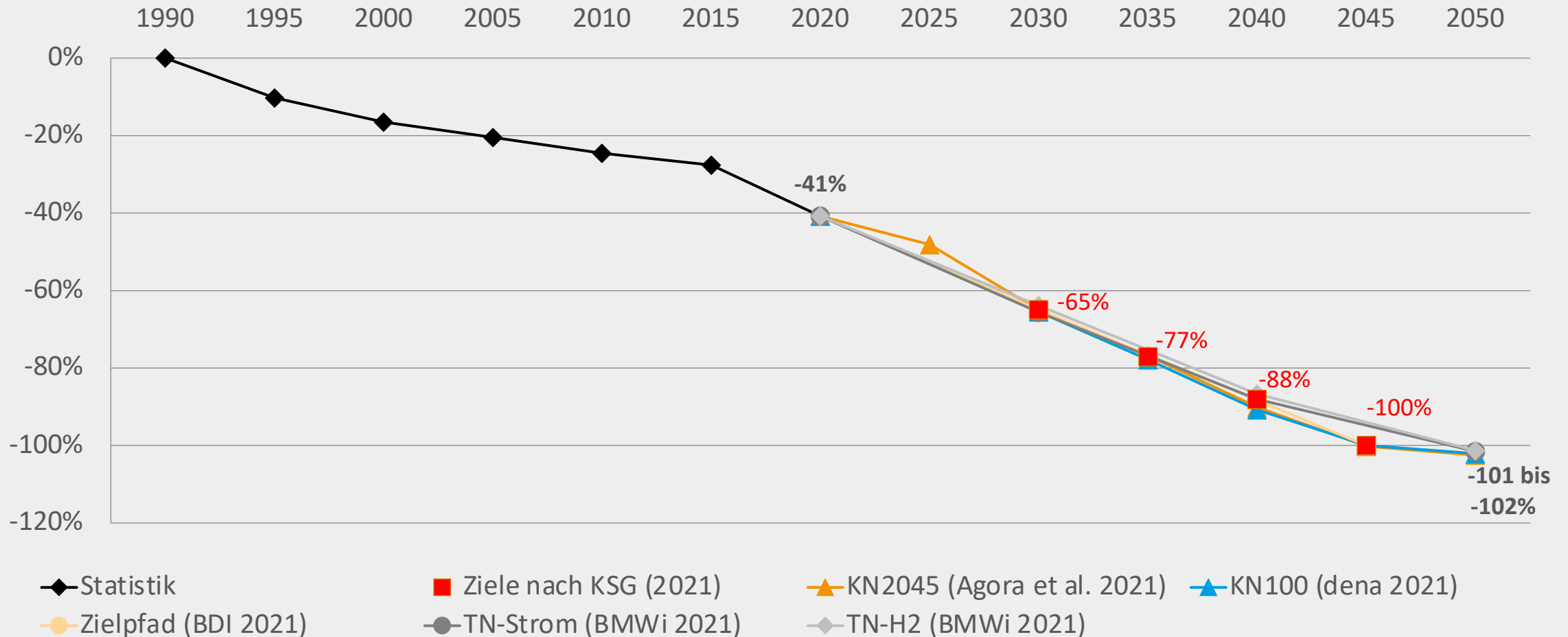
Änderung der gesamten deutschen Treibhausgasemissionen gegenüber 1990
