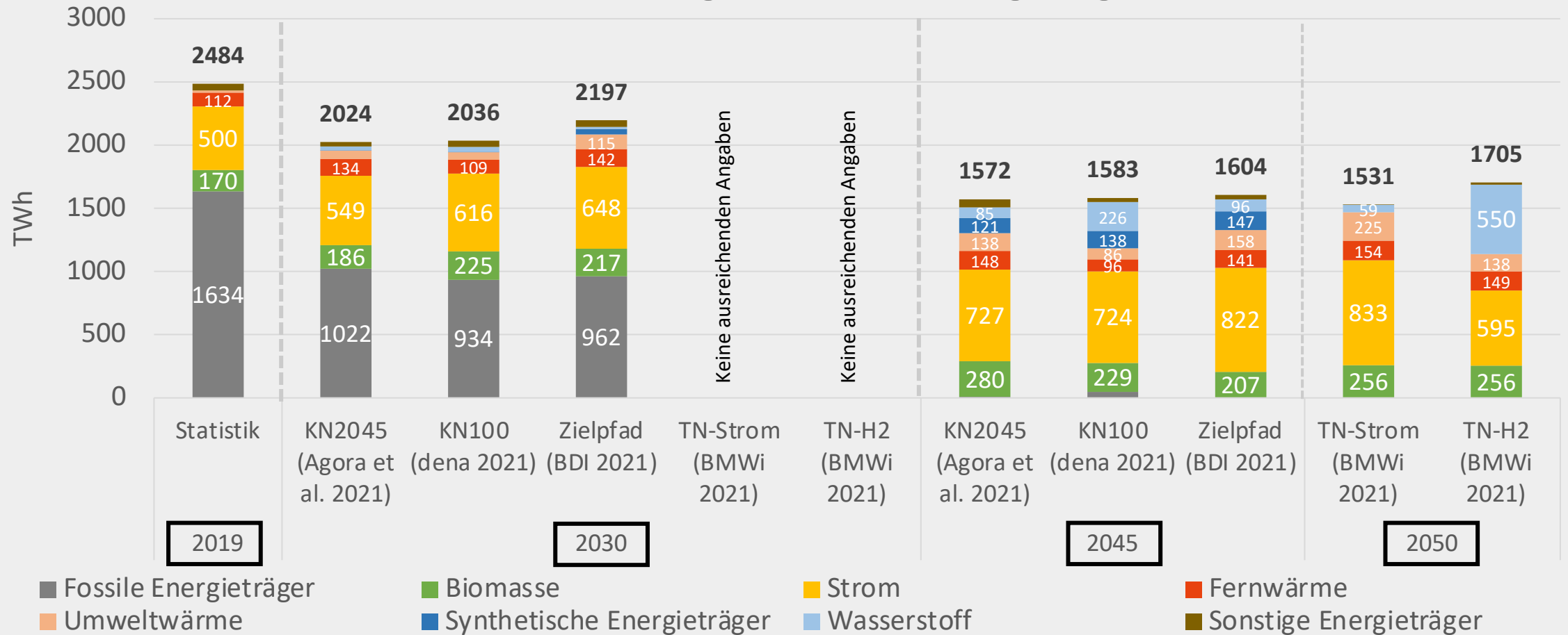
Gesamter Endenergiebedarf nach Energieträgern
