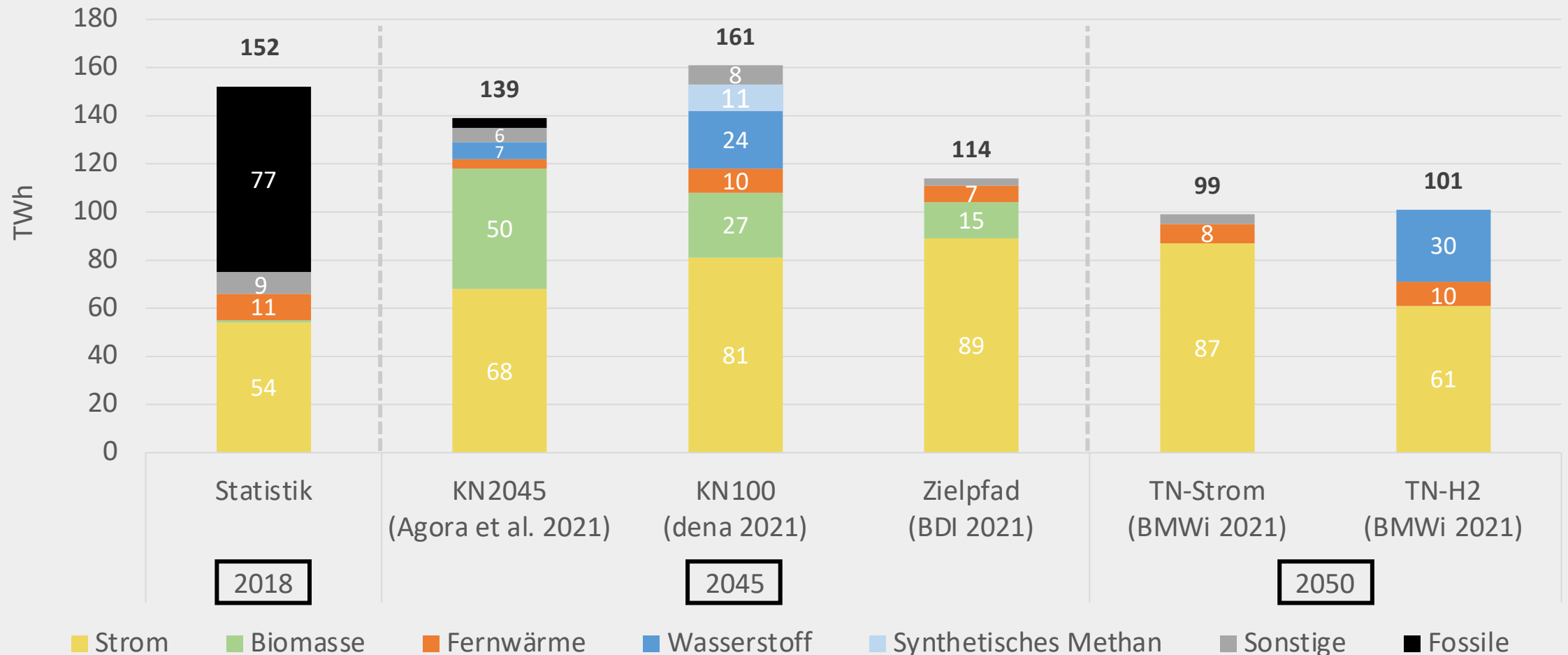
Endenergieverbrauch der chemischen Industrie nach Energieträgern
