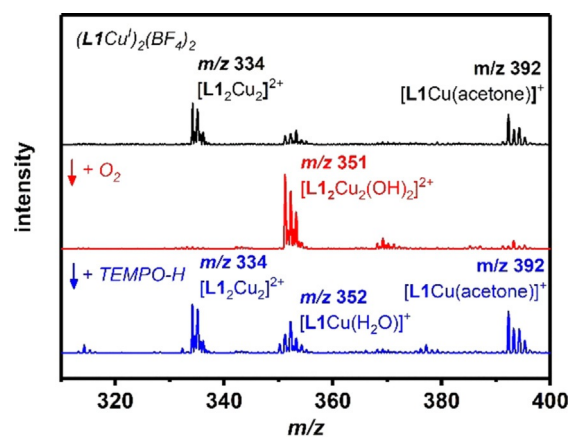
Abbildung 1. ESI-MS-Spektren von 1 in Aceton im positiven Modus mit Signalen von [\text{L}_1\text{Cu}_2]^{2+} ( m/z 334) und [\text{L}_1\text{Cu}(\text{acetone})]^+ ( m/z 392) (oben, schwarz); vom Reaktionsprodukt von 1 mit \text{O}_2 bei -10^\circ\text{C} mit Signalen von [\text{L}_1\text{Cu}_2(\text{OH})_2]^{2+} ( 3 ) bei m/z 351 gemischt mit Signalen von [\text{L}_1\text{Cu}(\text{OH})]^+ , [\text{L}_1\text{Cu}_2(\text{OH})(\text{F})]^{2+} und [\text{L}_1\text{Cu}(\text{F})]^+ (siehe Abbildung S5 für Dekonvolution) (mitte, rot); und die Produkte der Zugabe von TEMPO-H zu einer Lösung von 3 übereinstimmend mit den Kupfer(I)-Komplexen [\text{L}_1\text{Cu}_2]^{2+} ( m/z 334), [\text{L}_1\text{Cu}(\text{H}_2\text{O})]^+ ( m/z 352) und [\text{L}_1\text{Cu}(\text{acetone})]^+ ( m/z 392) (unten, blau).
