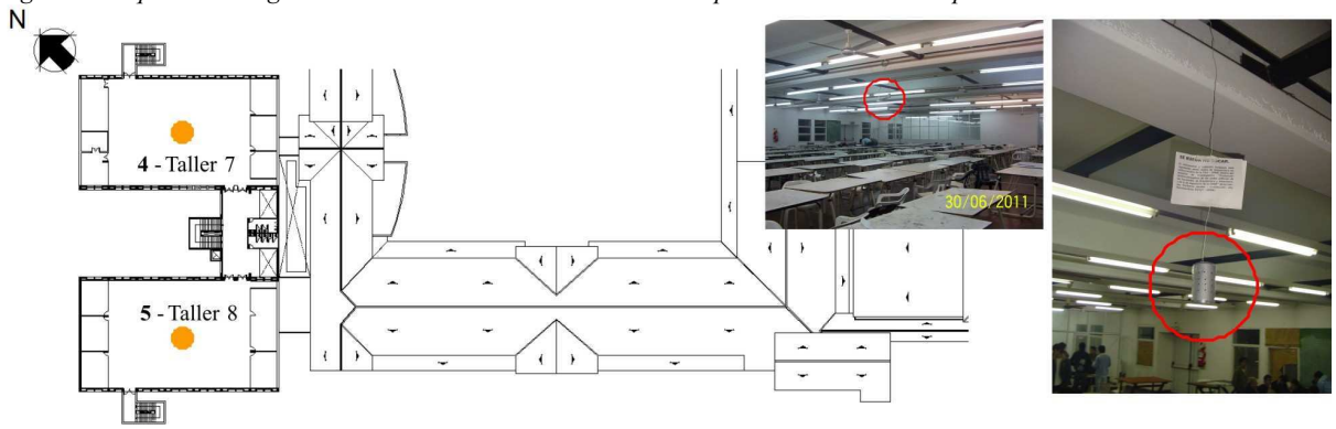
Figura 5: Esquema e imágenes de distribución de los sensores de temperatura en Planta 2º piso – FAU – UNNE.
