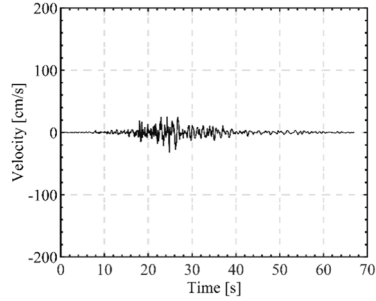
(d) HWA velocity time histories
