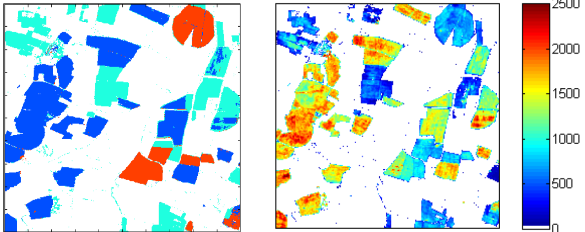
Figure 10 : A gauche : carte des cultures d'été (maïs (bleu), soja (rouge), tournesol (cyan)). A droite, carte des biomasses aériennes estimées à partir d'images FORMOSAT-2 et du modèle SAFY. La zone représentée mesure 500 sur 500 mètres et se situe près de Lamasquère [Claverie et al., soumis].
