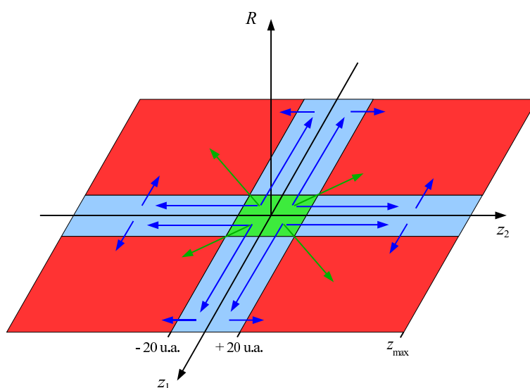
FIG. 4.8 – Schéma des différentes «zones» sur le plan (Oz_1z_2) à une distance internucléaire R donnée. En vert et au centre, est représentée la zone « \text{H}_2^+ ». Les bandes bleues, le long de chacun des axes z_1 et z_2 , illustrent les zones « \text{H}_2^+ ». Enfin, les carrés rouges symbolisent les zones « \text{H}^+ + \text{H}^+ ». Les flèches bleues représentent l'ionisation double séquentielle. Les flèches vertes symbolisent l'ionisation double non séquentielle (voir le chapitre 2 pour de plus amples détails).
