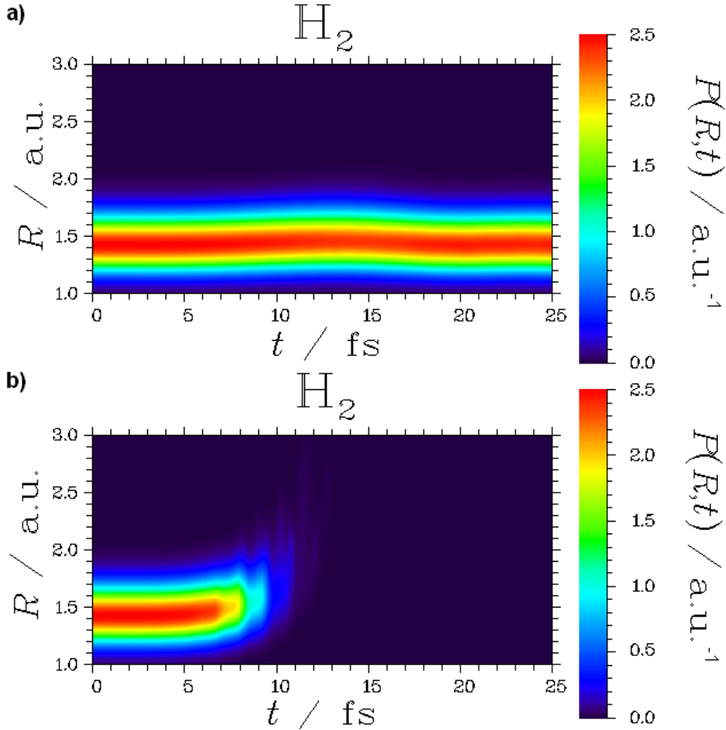
FIG. 5.3 – Densité de probabilité de H_2 en fonction de la distance internucléaire et du temps à des éclairements de a) I = 10^{14} \text{ W.cm}^{-2} et b) I = 8 \times 10^{14} \text{ W.cm}^{-2} pour une impulsion laser de durée 10 fs et une phase absolue \varphi = 0 .
