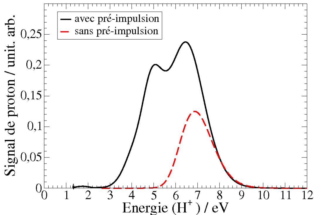
FIG. 6.5 – Spectres théoriques d'énergie cinétique des protons issus de l'impulsion de la figure 6.4 avec (en traits pleins noirs) et sans (en tirets rouges) la pré-impulsion à 10^{14} W.cm -2 .
