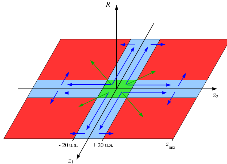
FIG. 7.4 – Schéma des différentes «zones» sur le plan (Oz_1z_2) à une distance internucléaire R donnée. En vert et au centre, est représentée la zone «H 2 ». Les bandes bleues, le long de chacun des axes z_1 et z_2 , illustrent les zones «H 2 + ». Enfin, les carrés rouges symbolisent les zones «H + + H + ». Les flèches bleues représentent l'ionisation double séquentielle. Les flèches vertes symbolisent l'ionisation double non séquentielle.
