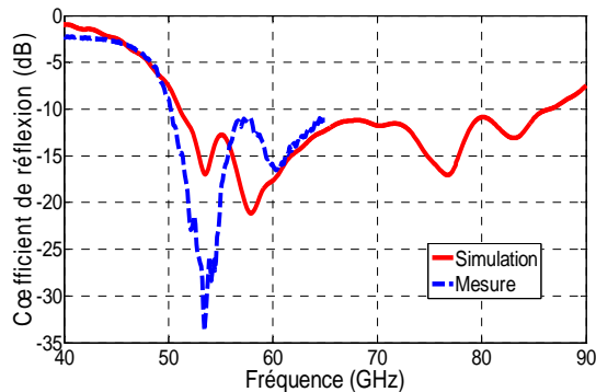
Figure 7 : Effet de structure d'alimentation sur S_{11}
