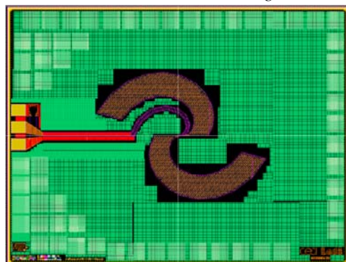
Figure 6 : Schématisation de l'antenne double spirale avec dummies après cadence ®
