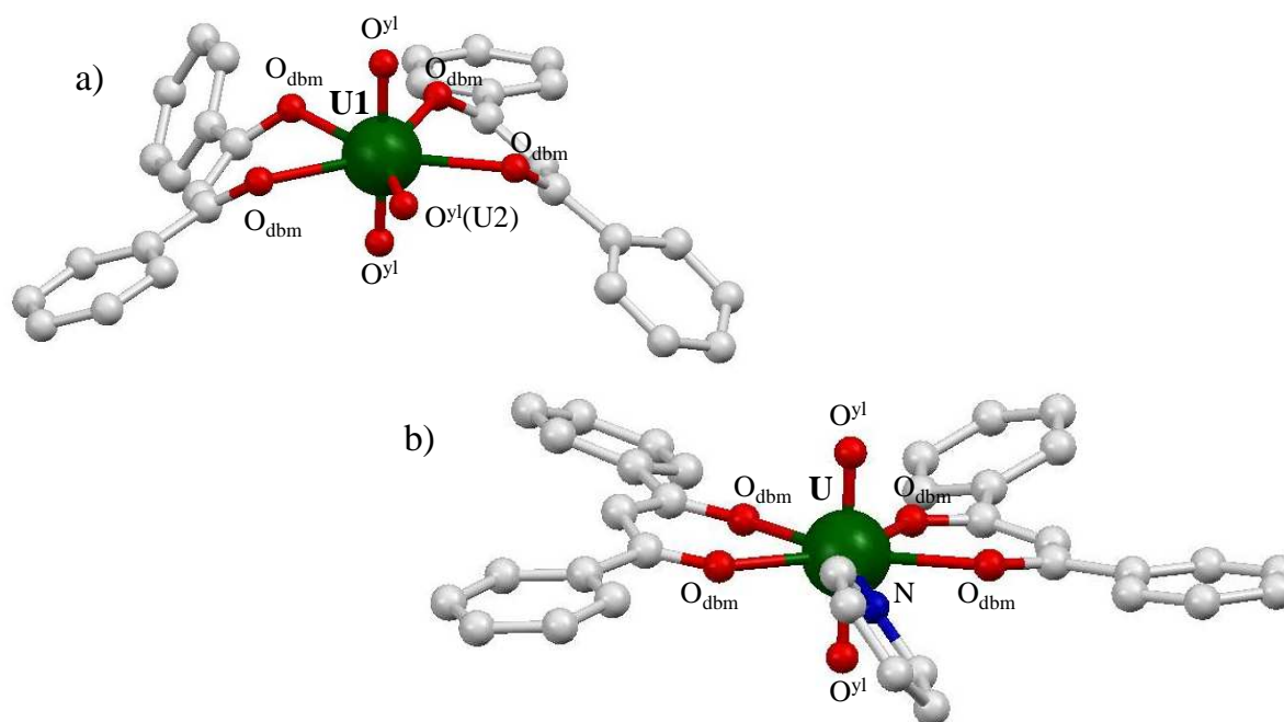
Figure III.4 : Comparaison structurale a) du motif [\text{UO}_2]^+ du tétramère \{[\text{UO}_2(\text{dbm})_2]_4[\text{K}_4(\text{CH}_3\text{CN})_4]\} ( 13 ) et b) du complexe [\text{UO}_2(\text{dbm})_2\text{py}] . 13 Les atomes d'hydrogènes ont été omis pour des raisons de clarté.
