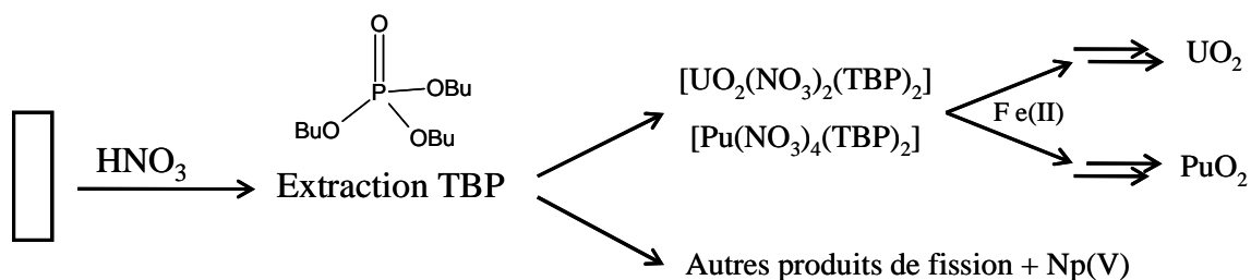
Figure I.3 : Schéma de principe du procédé PUREX.
