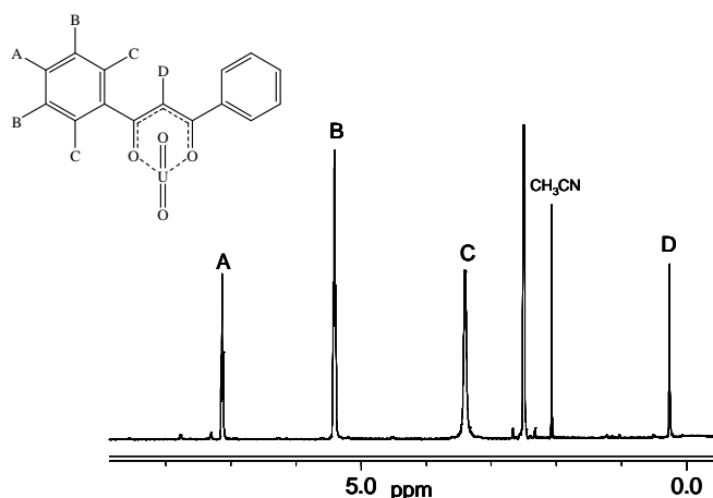
Figure III.18 : Spectre RMN ^1\text{H} à 400 MHz et 298K du complexe 13 dans le \text{dmsO-d}_6 ( C = 1,6 \text{ mM} ).
