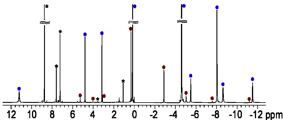
Figure III.30 : Spectre RMN ^1\text{H} à 400 MHz et 298K du complexe 15 dans la pyridine- d_5 (au dessus) et représentation des deux isomères 1 et 2 (en dessous). (*, solvants et impuretés)
