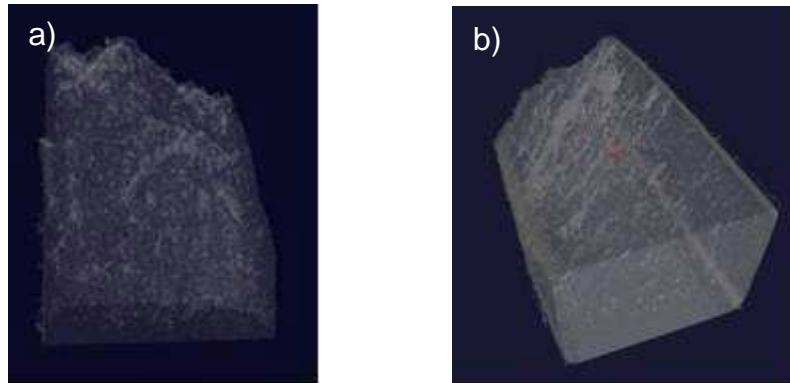
Figure 8. Rendus volumiques 3D. a) éprouvette sollicitée en sens axial ; b) éprouvette sollicitée en sens circonférentiel.
