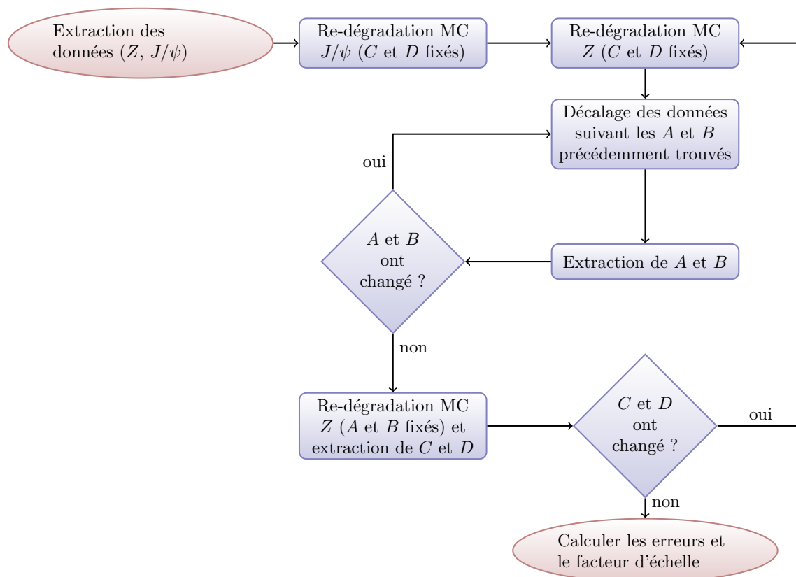
FIGURE 5.18 – L'organigramme de l'algorithme itératif implémenté afin d'obtenir les meilleurs paramètres de dégradation des muons.
