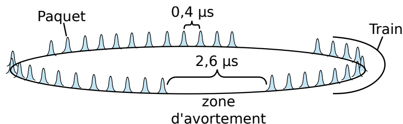
FIGURE 2.9 – Schéma illustrant la répartition des paquets de protons et d'antiprotons dans le Tevatron avec les temps de séparation.
