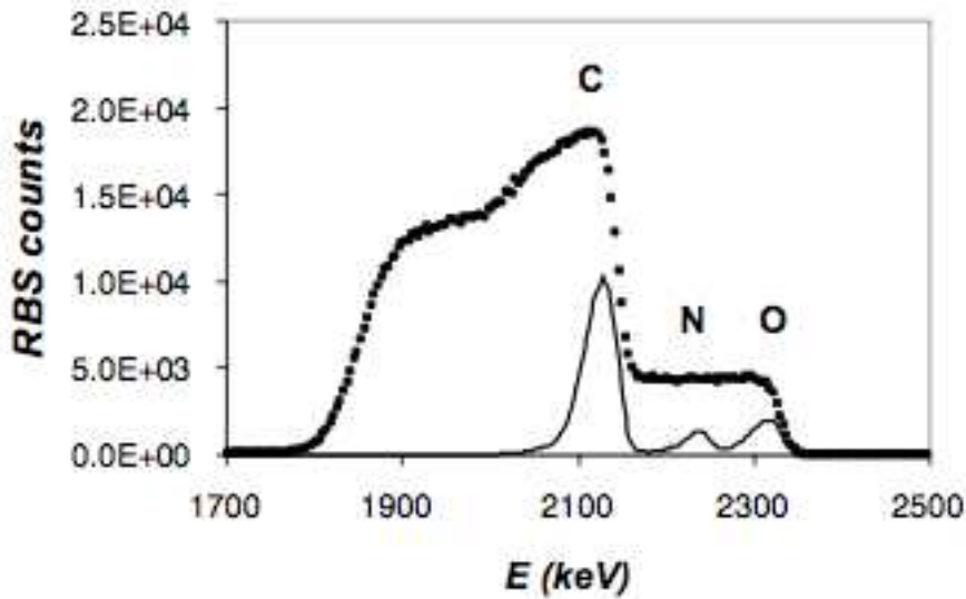
FIGURE 5.1: Spectres RBS du support polymère seul (points) et du tapis cellulaire seul (traits)
