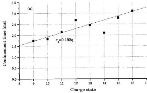
FIGURE 2.5: Temps de confinement dans un plasma d'argon avec P RF = 1100 W, déduits des mesures de densités et courants ioniques.
