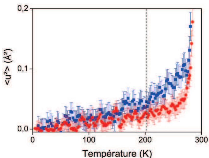
Figure 6-2. Evolution du déplacement carré moyen \langle u^2 \rangle avec la température de la myoglobine libre (■) et adsorbée (●) sur les NP de silice 7 nm dans une solution de D_2O (13% en masse Mb, 30% en masse NP), mesurée par diffusion incohérente de neutrons. Les pointillés marquent la transition dynamique de la myoglobine libre que l'on observe peu après 200 K.
