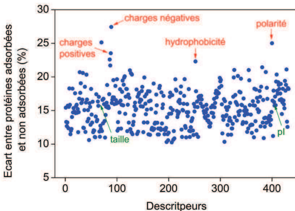
Figure 4-22. Ecart entre la valeur moyenne de chacun des 432 critères testés par le programme Profestat (66) entre protéines de levure adsorbées et non adsorbées (%). La différence est exprimée en valeur absolue et reflète aussi bien un enrichissement qu'un appauvrissement dans les protéines adsorbées par rapport aux non adsorbées. Quelques exemples de critères différents (en rouge) et semblables (en vert) entre les deux groupes sont donnés.
