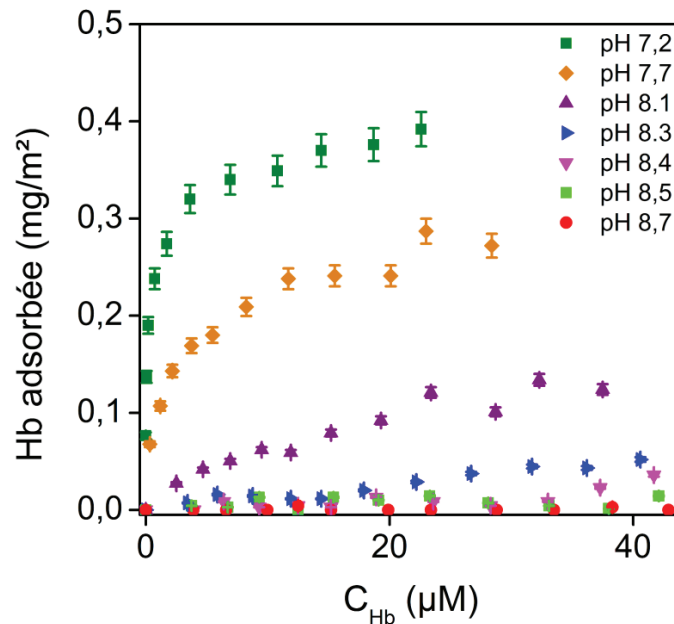
Figure 4-10. Isothermes d'adsorption de l'hémoglobine sur les nanoparticules de silice 20 nm en tampon Tris-HCl 100 mM en fonction du pH
