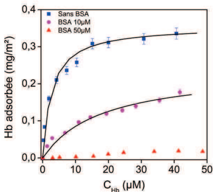
Figure 4-17. Isothermes d'adsorption de l'hémoglobine sur les NP de silice 20 nm en tampon Phosphate 100 mM à pH 7,4 pour différentes concentrations initiales en BSA : 0 ( \blacksquare ), 10 \mu\text{M} ( \blacksquare ) et 50 \mu\text{M} ( \blacktriangle ) ; modèle de Langmuir (en noir). Les NP sont mises en contact avec la BSA puis l'hémoglobine est ajoutée à la solution contenant BSA et NP ( C_{\text{NP}} = 4,5 \text{ mg/mL} )
