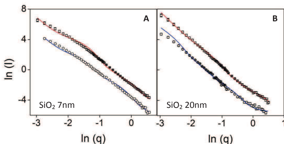
Figure 3-7. Profils d'intensité mesurés en diffusion de neutrons aux petits angles sur NP SiO 2 7 nm (A) et sur NP SiO 2 20 nm (B) sur poudre (■) et en suspension à 30 mg/mL dans D 2 O (●); modélisation par une distribution de particules sphériques (courbe rouge sur poudre, courbe bleue en suspension)
