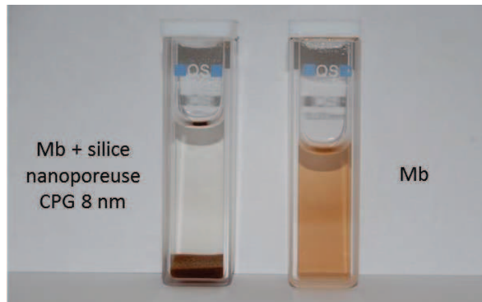
Figure 4-2. Photographie d'une solution de myoglobine libre ( C_{Mb} = 40 \mu M ) (à droite) et en présence de silice nanoporeuse CPG 8 nm ( m = 150 \text{ mg} ) (à gauche) en tampon Phosphate 100 mM à pH 7,4 après décantation des particules
