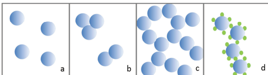
Figure 3-9. Interactions possibles entre nanoparticules en solution : (a) suspension, (b) agrégats, (c) gel, (d) agrégation par adsorption de protéines (en vert) d'après (25)
