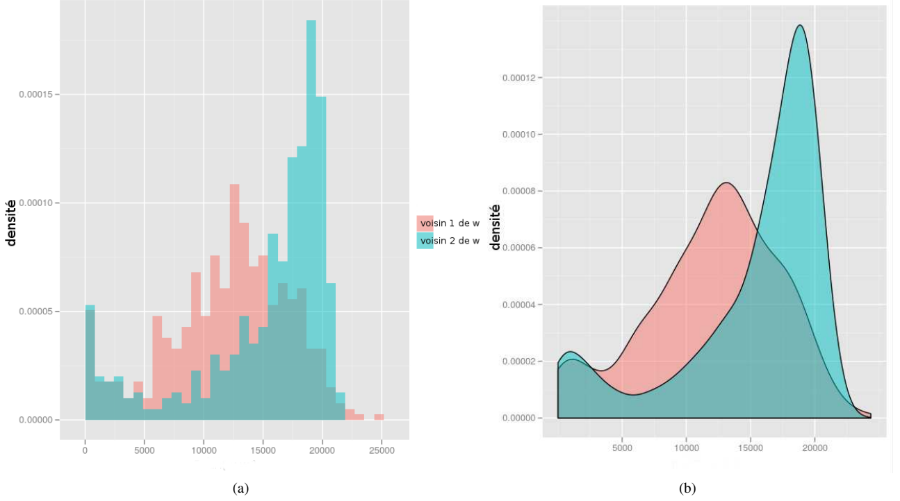
FIGURE 2: (a) Deux histogrammes (en bleu et en rouge) des écarts d'un mot et deux de ses voisins. (b) Deux densités de probabilités (en bleu et en rouge) estimées par fenêtres de Parzen, correspondant aux données de la figure 2a.
