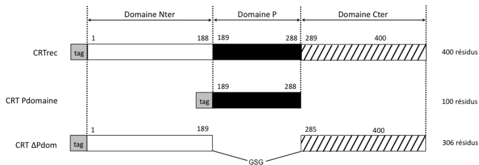
Figure 23 : Schéma représentatif des différents domaines disponibles de la calréticuline humaine recombinante
