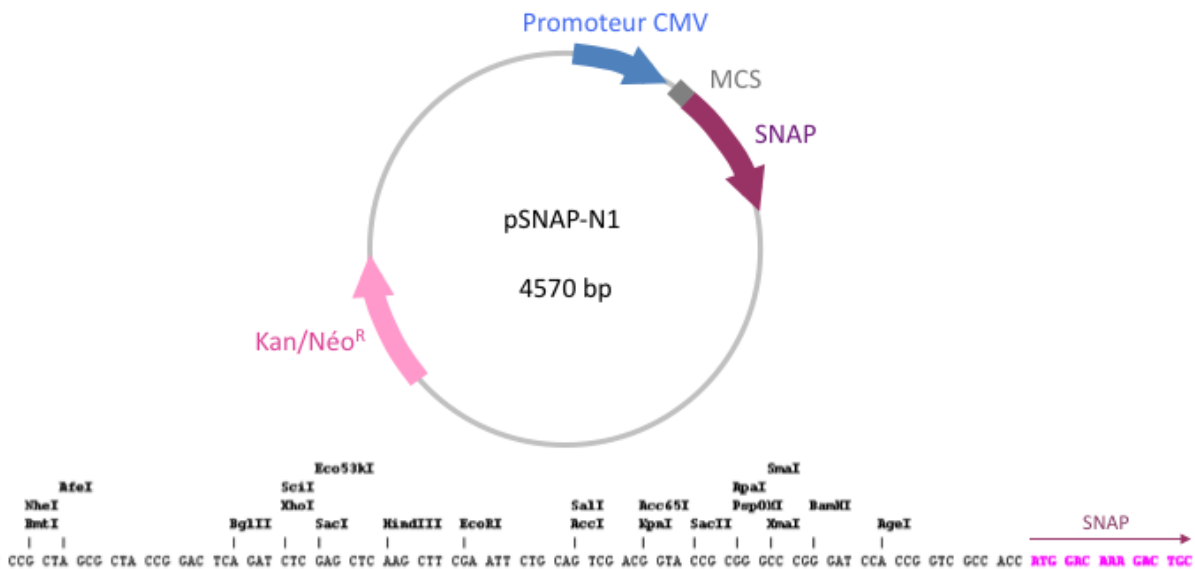
Figure 90 : Schéma de la carte du plasmide pSNAP-N1
