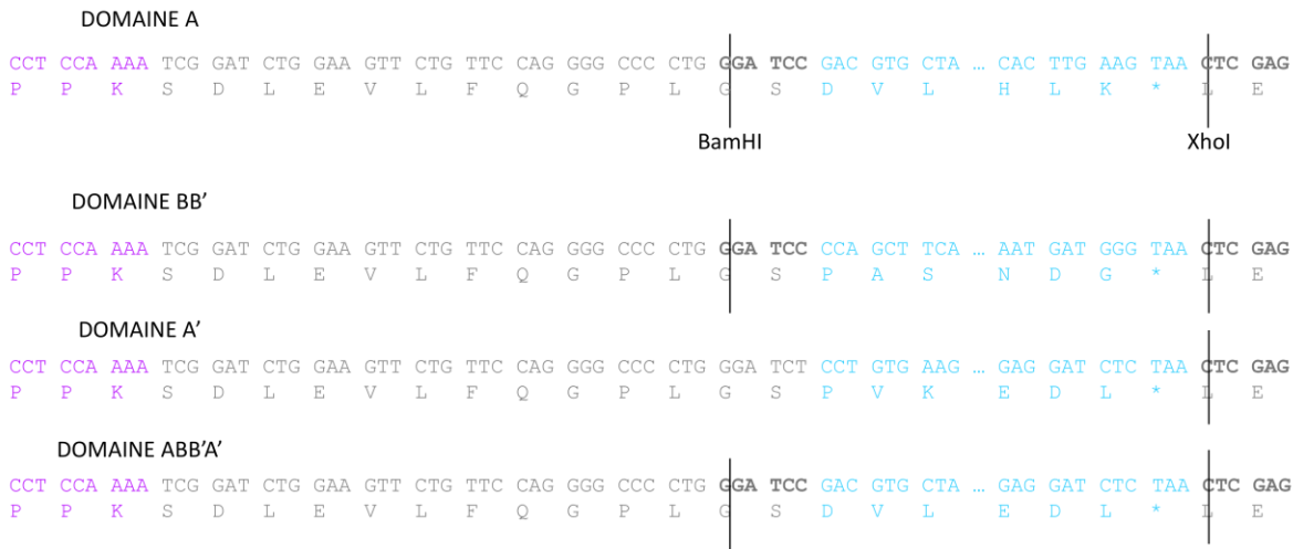
Figure 94 : Séquence du plasmide pGEX-ERp57 en fonction de différents domaines clonés au niveau des sites de restriction BamHI et XhoI
