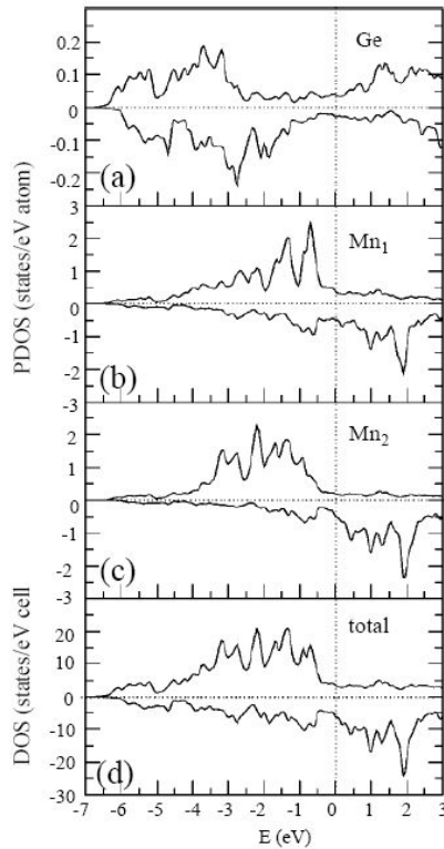
Fig. I-7 : densité d'états projetée sur les trois types d'atome composant le Mn_5Ge_3 (a) – (c), et densité d'états totale (d) [Picozzi04].
