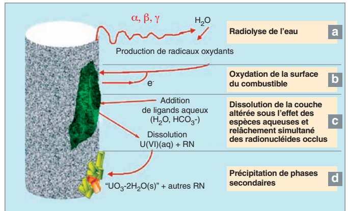
Fig. 90. Mécanismes génériques d'altération d'un combustible nucléaire usé en présence d'eau : (a) radiolyse de l'eau sous l'effet des rayonnements \alpha , \beta ou \gamma , (b) oxydation de la surface du combustible et transformation de U(IV) en U(VI), (c) dissolution de la couche altérée sous l'effet des espèces aqueuses et relâchement simultané des radionucléides occlus, (d) précipitation le cas échéant de phases secondaires.
