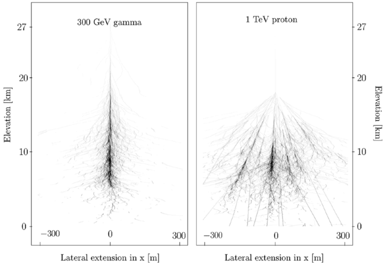
FIGURE 4.2: Simulations d'une gerbe EM de 300 GeV et d'une gerbe hadronique initiée par un proton de 1 TeV (Crédits : [Aharonian et al., 2008]).
