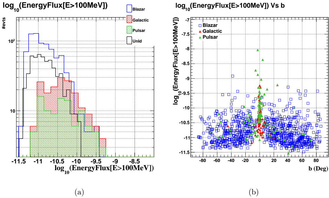
FIGURE 10.1: Propriétés des sources identifiées et non-identifiées. (a) Distribution du flux d'énergie entre 0,1 et 100 GeV des blazars (bleu), des sources galactiques (rouge), des pulsars (vert) et de l'ensemble des source non-identifiées (noir). (a) Flux d'énergie en fonction de la latitude galactique pour les blazars (bleu), les sources galactiques (rouge) et les pulsars (vert).
