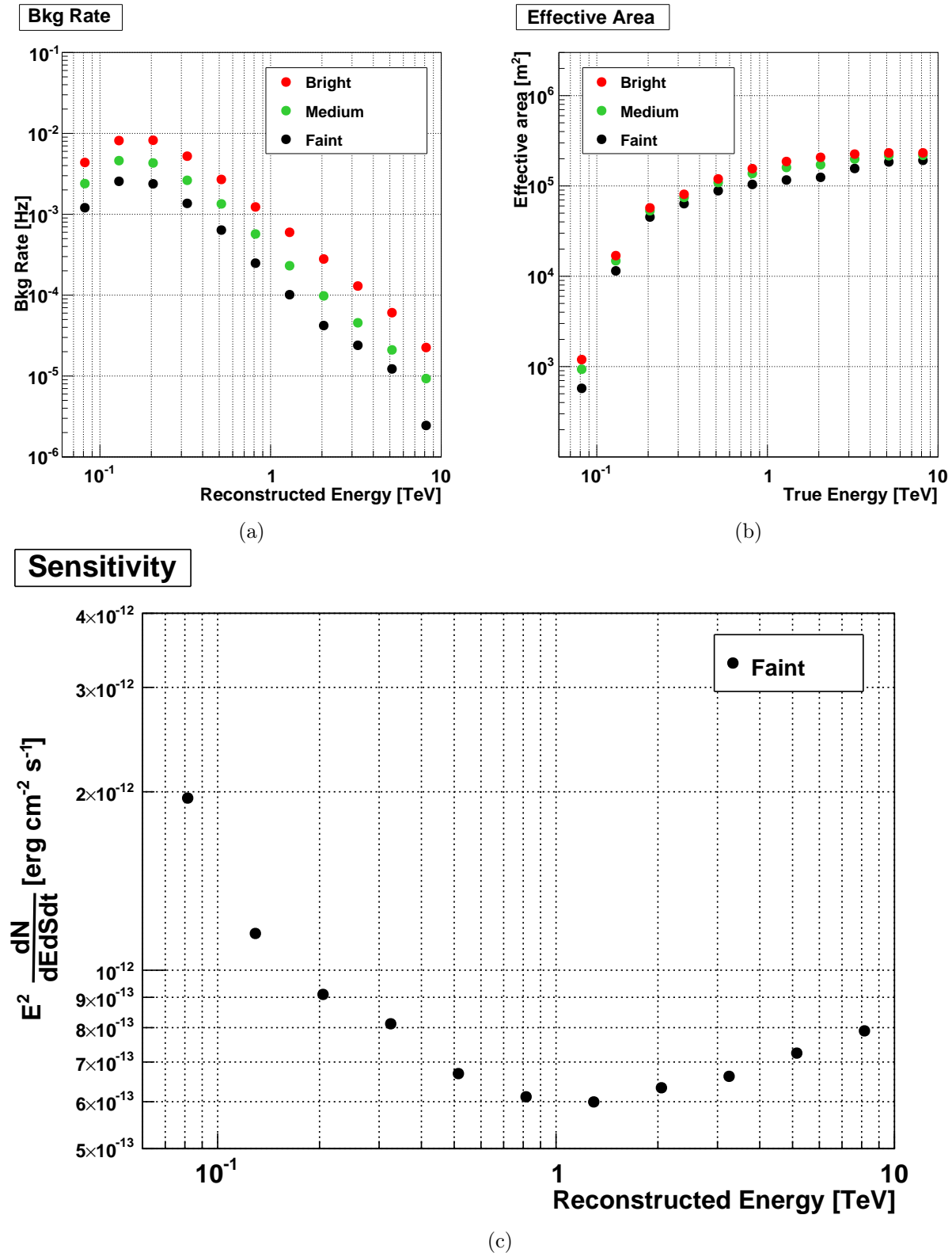
FIGURE 7.3: (a) Taux de fond en fonction de l'énergie reconstruite pour les trois configurations. (b) Surface efficace de collection en fonction de l'énergie vraie pour les trois configurations. (c) Sensibilité différentielle en fonction de l'énergie reconstruite de la configuration dédiée à l'étude des sources faibles pour un temps d'observation de 50 h et pour une détection à 5\sigma dans chaque intervalle d'énergie reconstruite.
