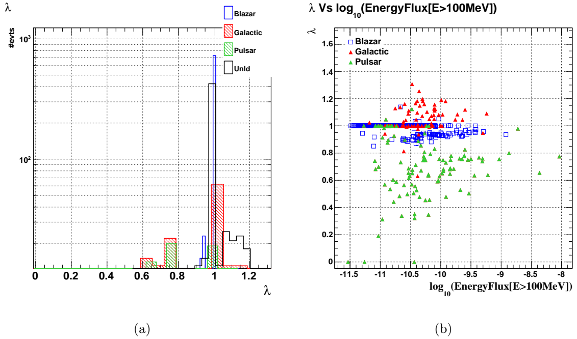
FIGURE 10.2: (a) Distribution de paramètre \lambda et (b) ses corrélations avec le flux en énergie ( E > 100 MeV).
