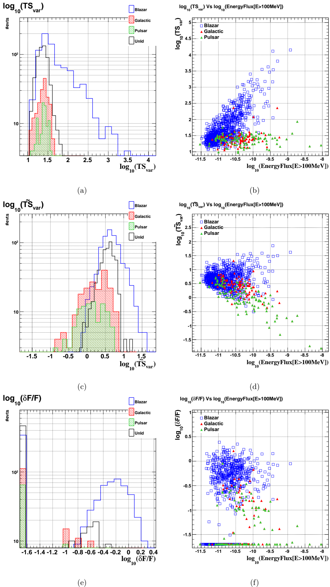
FIGURE 10.6: (a) – (c) Distributions des paramètres TS_{var} , \tilde{TS}_{var} et \delta F/F . (b) – (d) et (f) leurs
