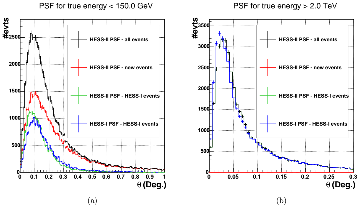
FIGURE 6.1: Précision angulaire obtenue avec la méthode des ellipses pour différents lots d'événements vus par le réseau de 5 télescopes, ayant une énergie vraie (a) inférieure à 150 GeV et (b) supérieure à 2 TeV. Les distributions verte et rouge représentent les deux populations définies dans le texte : les événements déjà observés par le réseau HESS-I et les événements de multiplicité deux ayant déclenché CT_5 . La distribution noire représente la somme de ces deux lots d'événements. Quant à la distribution bleue, elle représente la précision angulaire obtenue avec les événements déjà détectés en mode stéréo pour lesquelles on a supprimé CT_5 de la reconstruction. Sur la sous-figure (b), les événements de multiplicité deux ayant déclenché CT_5 représentent une fraction négligeable ( <0,1\% ) de l'ensemble des événements vus par le réseau (la courbe verte et la courbe noire sont quasiment confondues).
