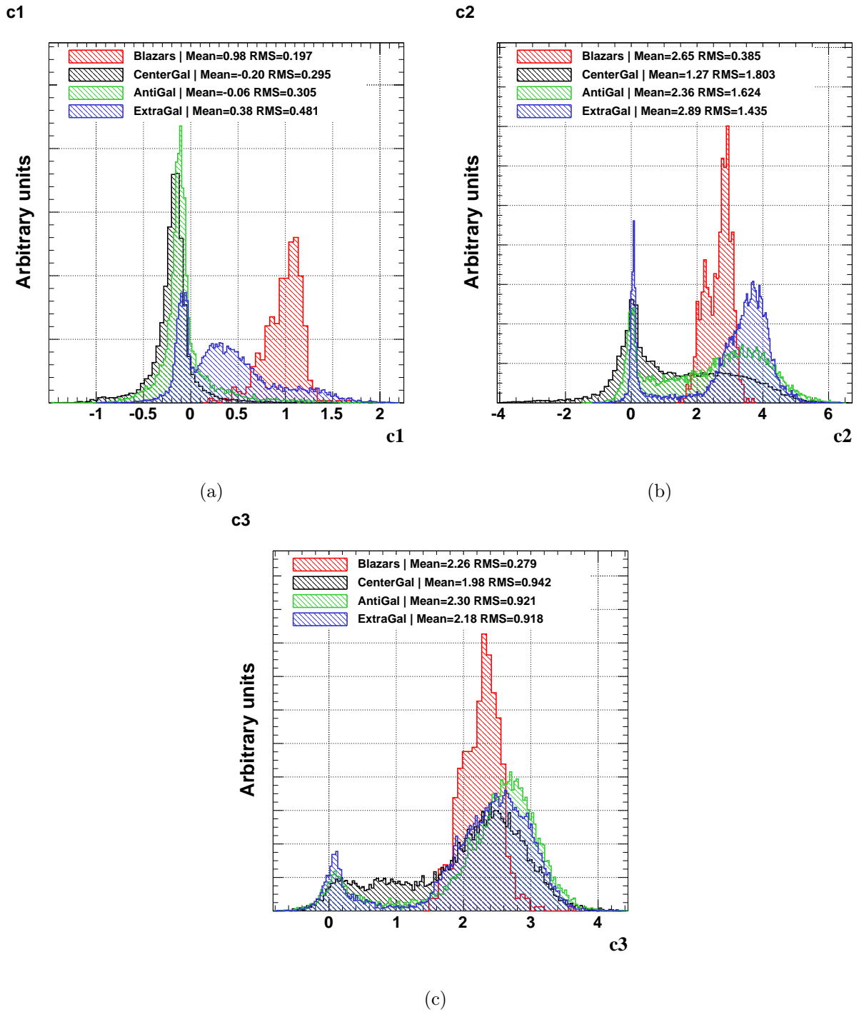
FIGURE 11.5: Distributions des couleurs c_1 , c_2 et c_3 obtenues après correction de l'extinction infra-rouge (voir texte) pour les sources possédant un niveau de signal sur bruit supérieur à 5 dans les trois premiers filtres et supérieur à 3 dans le dernier filtre. Les différents histogrammes représentent les blazars identifiés (rouge), le fond « extragalactique » (bleu), le fond « centre galactique » (noir) et le fond « anti-centre galactique » (vert).
