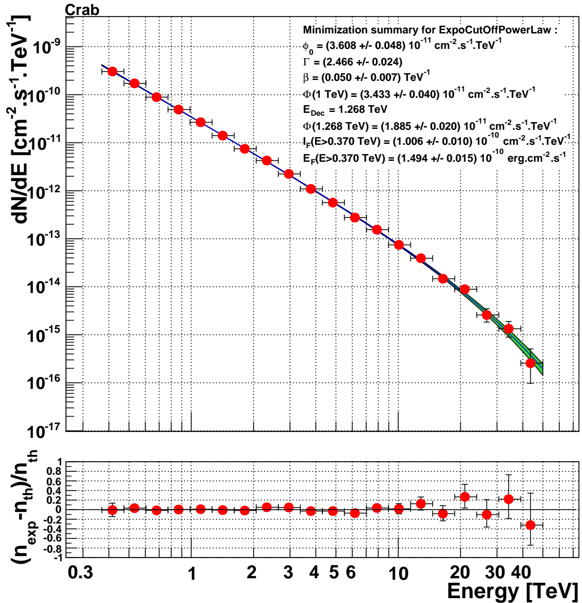
FIGURE 5.20: Spectre de la nébuleuse du Crabe avec une hypothèse de loi de puissance avec une coupure exponentielle généré avec START pour un temps d'observation effectif de 43,8 h ( N_{\sigma} \approx 168 ).
