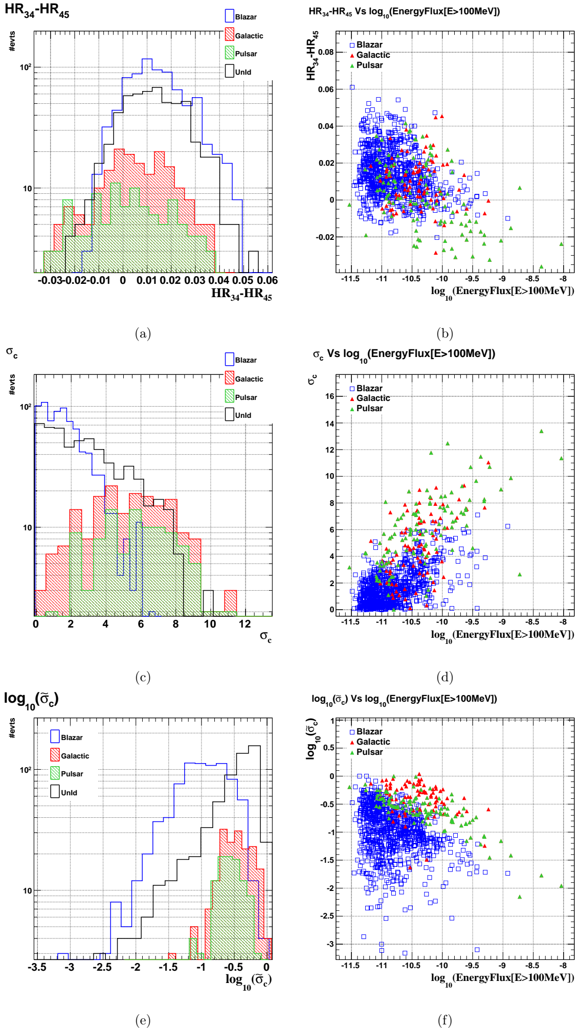
FIGURE 10.5: (a) (c) (e) Distributions des paramètres HR_{34} - HR_{45} , \sigma_c et \tilde{\sigma}_c (b) (d) et (f) leurs
