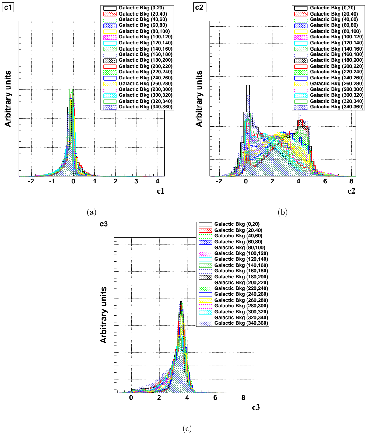
FIGURE 11.3: Variation spatiale des distributions des couleurs c_1 , c_2 et c_3 pour le fond infrarouge galactique. Les différents histogrammes représentent les contributions infrarouges de 18 régions du centre galactique correspondant à autant de tranches de largeur de 20^\circ en longitude. Les bornes en longitude de chaque tranche sont indiquées.
