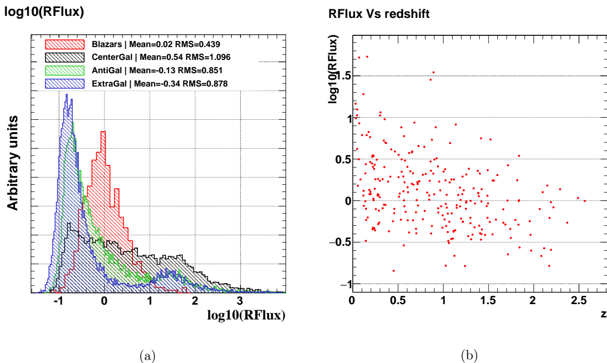
FIGURE 11.6: (a) Distributions du paramètre RFlux obtenues après correction de l’extinction infrarouge (voir texte) pour les sources possédant un niveau de signal sur bruit supérieur à 5 dans les trois premiers filtres et supérieur à 3 dans le dernier filtre. Les différents histogrammes représentent les blazars identifiés (rouge), le fond « extragalactique » (bleu), le fond « centre galactique » (noir) et le fond « anti-centre galactique » (vert). (b) Paramètre RFlux en fonction du redshift pour les blazars identifiés dont le redshift est connu.
