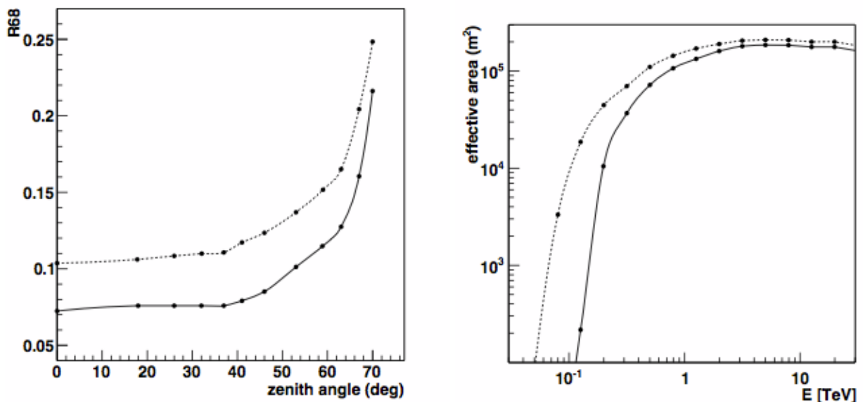
FIGURE 5.15: (a) Précision angulaire à 68% en fonction de l'angle zénithal pour un offset de 0,5° et (b) surface efficace de collection en fonction de l'énergie vraie de l'analyse Paris-MVA à un angle zénithal de 18°, pour deux configurations d'analyse qui sélectionnent les images avec un seuil en charge de 40 p.e. (traits pointillés) et de 150 p.e. (traits pleins) [Becherini et al., 2011].
