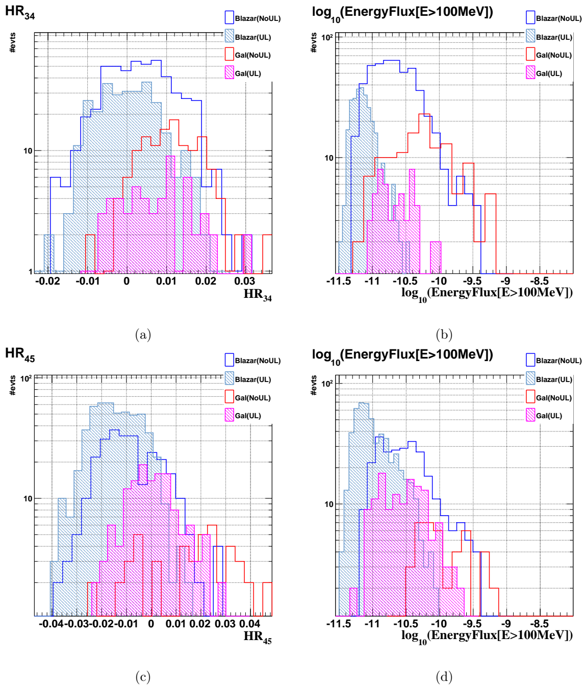
FIGURE 10.11: Stabilité des indices de duretés HR_{34} et HR_{45} selon la présence de limite supérieur dans le calcul. À gauche distributions des paramètres HR_{34} et HR_{45} (bleu=blazars sans limite supérieure, bleu hachuré=blazars avec au moins une limite supérieure, rouge=sources galactiques sans limite supérieure, magenta hachuré=sources galactiques avec au moins une limite supérieure) et à droite distributions du flux en énergie des blazars et des sources galactiques (même code couleur).
