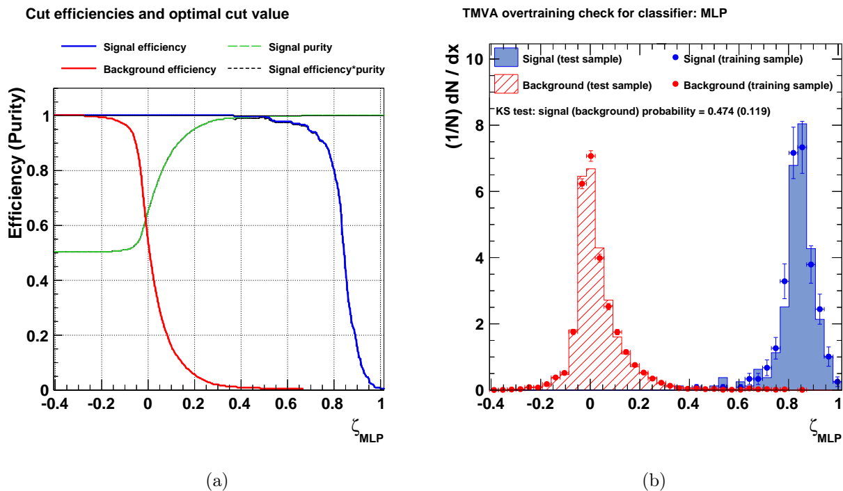
FIGURE 11.10: (a) Efficacités de reconstruction du signal (bleu) et du fond (rouge) en fonction de \zeta pour l'analyse « centre galactique ». (b) Distributions du paramètre \zeta des événements signal (bleu) et des événements de fond (rouge) pour les lots d'entraînement (traits pleins) et de test (points).
