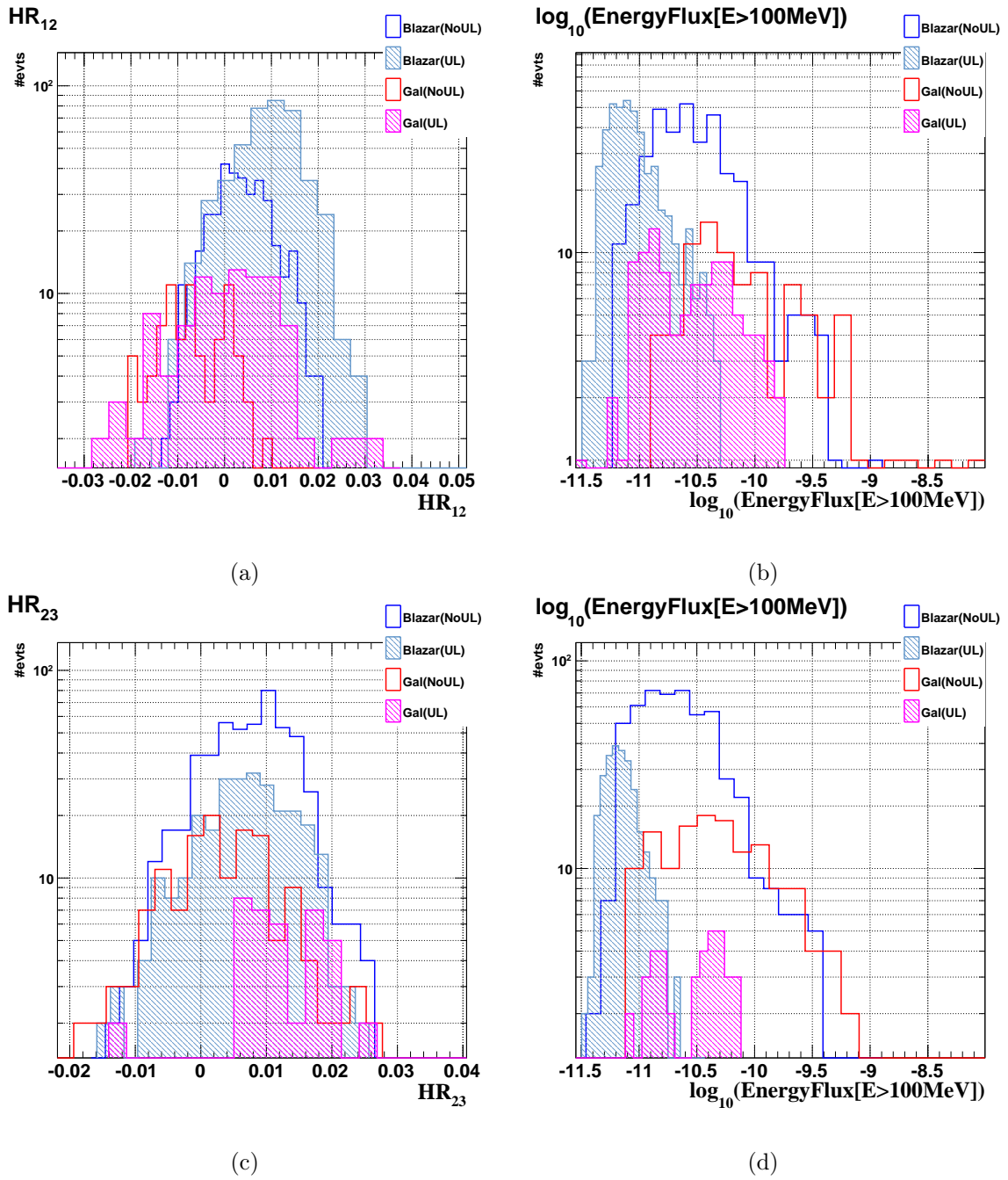
FIGURE 10.10: Stabilité des indices de duretés HR_{12} et HR_{23} selon la présence de limite supérieur dans le calcul. À gauche distributions des paramètres HR_{12} et HR_{23} (bleu=blazars sans limite supérieure, bleu hachuré=blazars avec au moins une limite supérieure, rouge=sources galactiques sans limite supérieure, magenta hachuré=sources galactiques avec au moins une limite supérieure) et à droite distributions du flux en énergie des blazars et des sources galactiques (même code couleur).
