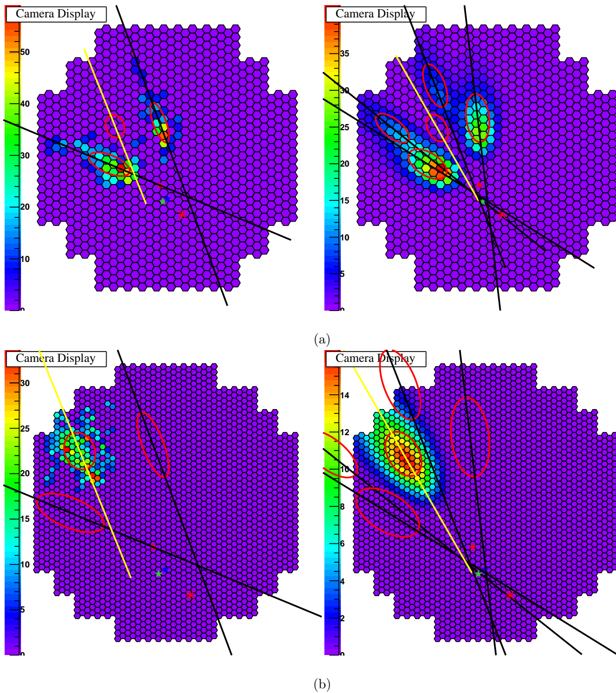
FIGURE 6.7: Illustration de la pré-sélection « modèle 3D » avec un proton simulé de 4,0 TeV. (a) À gauche, images mesurées passant la pré-sélection et projetées dans une caméra unique de type HESS-I. À droite, prédictions obtenues à partir de la projection de la photosphère et passant la pré-sélection « modèle 3D ». Les étoiles rouge, verte et bleue représentent respectivement les directions reconstruites avec les images mesurées passant la pré-sélection, les images projetées à partir du modèle et passant la pré-sélection « modèle 3D » et la direction provenant directement de l'ajustement du modèle 3D. L'astérisque rouge représente la direction vraie du proton. (b) Même chose que précédemment mais cette fois dans le référentiel de la cinquième caméra.
