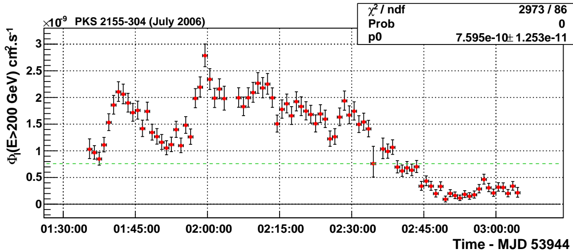
FIGURE 5.21: Exemple de courbe de lumière de la source PKS 2155-304 générée avec START. État haut observé lors de la nuit du 28 juillet 2006.
