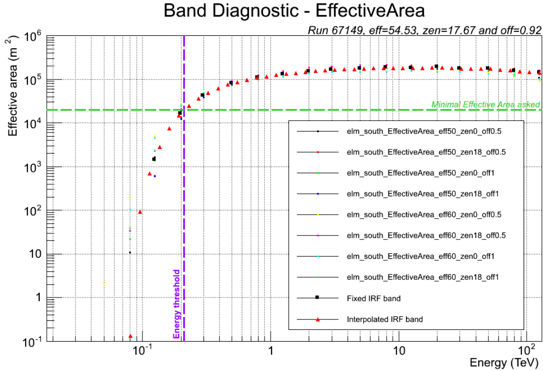
FIGURE 5.19: Surface efficace associée à un « run » d'observation.
