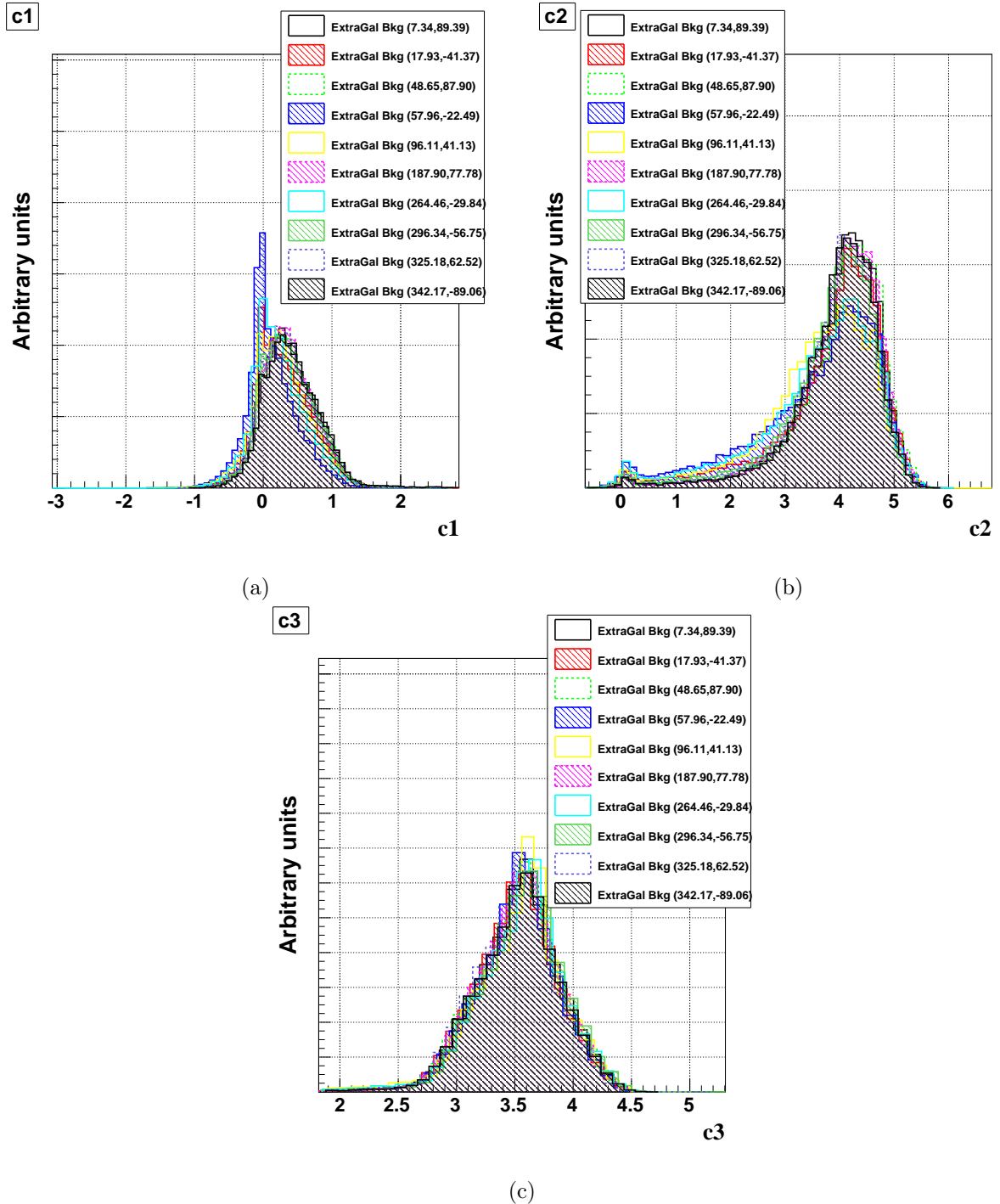
FIGURE 11.2: Variation spatiale des distributions des couleurs c_1 , c_2 et c_3 pour le fond infrarouge extragalactique. Les différents histogrammes représentent les contributions infrarouges de 10 régions extra-galactiques d'un rayon de 0,7^\circ tirées aléatoirement. Les coordonnées galactiques du centre de chaque région sont indiquées.
