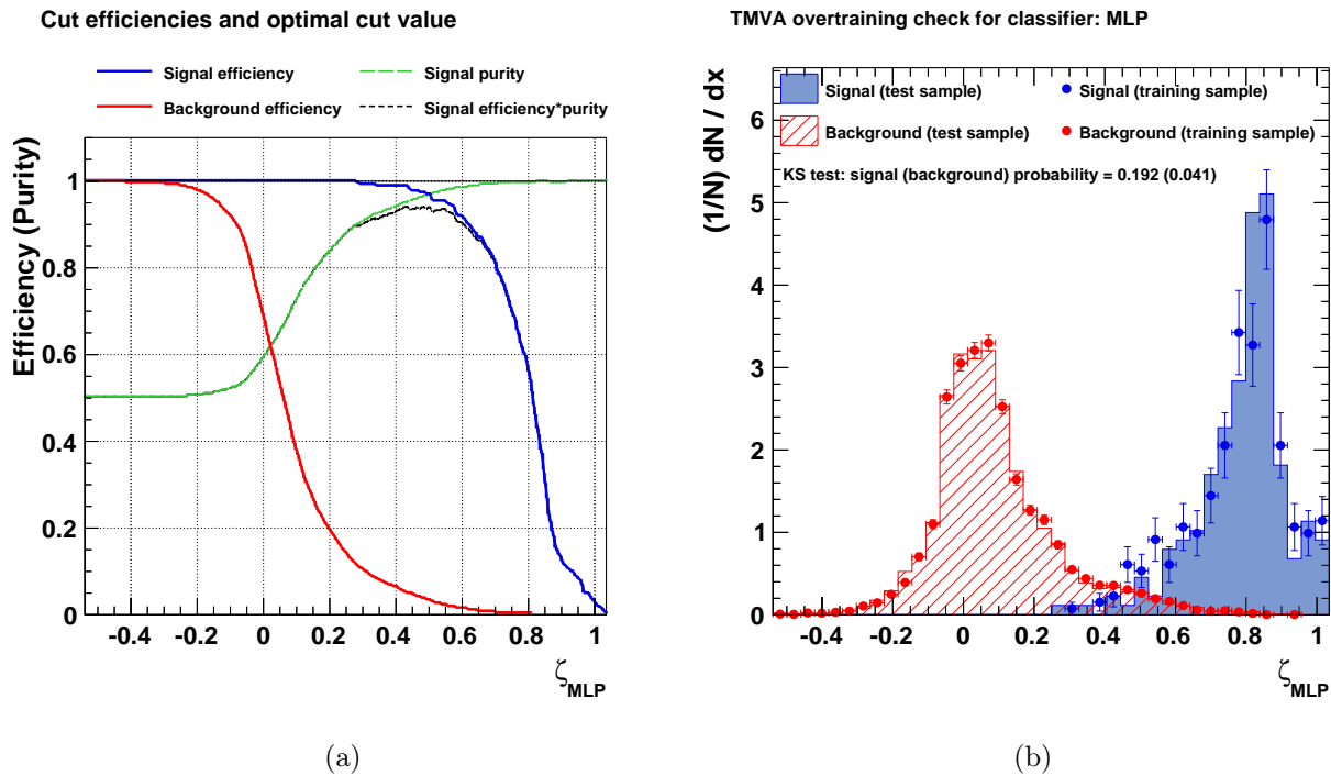
FIGURE 11.9: (a) Efficacités de reconstruction du signal (bleu) et du fond (rouge) en fonction de \zeta pour l'analyse « extragalactique ». (b) Distributions du paramètre \zeta des événements signal (bleu) et des événements de fond (rouge) pour les lots d'entraînement (traits pleins) et de test (points).
