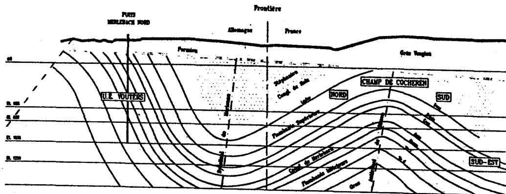
Figure 1 : Section of the Houillères du Bassin de Lorraine coalfield
