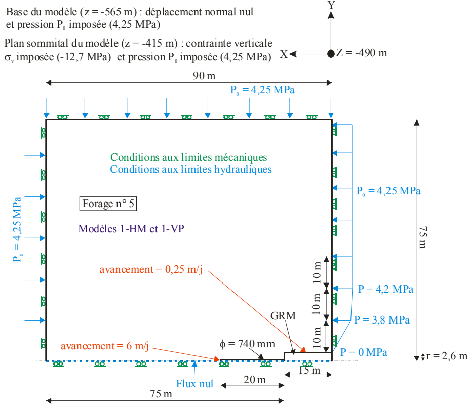
Figure 2 : Forage n° 5 dans la galerie GRM : géométrie et conditions aux limites.
