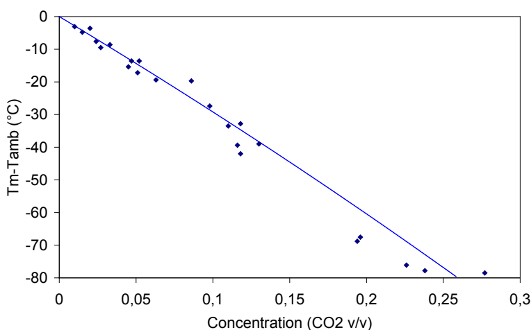
Figure 9 : Variations de température en fonction des concentrations CO 2 obtenues à l'aide de la mesure O 2
