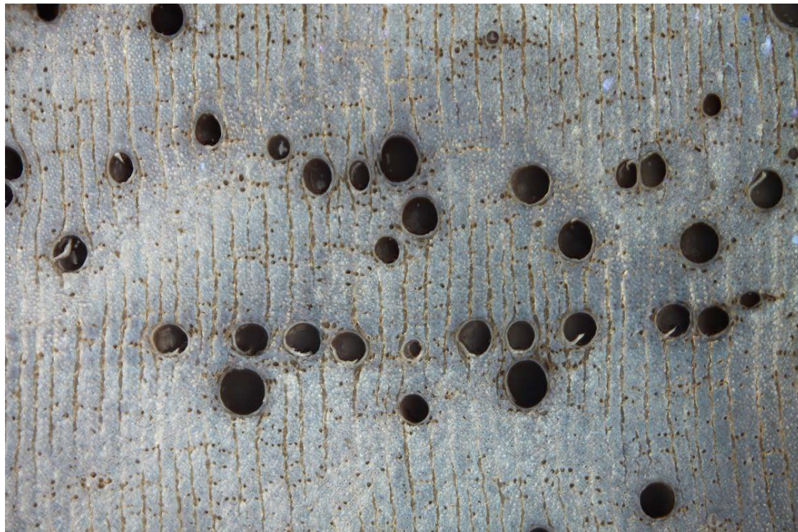
Figure 4 : microphotographie de la coupe transversale du bois du poteau de Baie-aux- Prunes (dimensions réelles 2,2 x 1,5 mm), Saint- Martin, cliché J. Beauchêne
