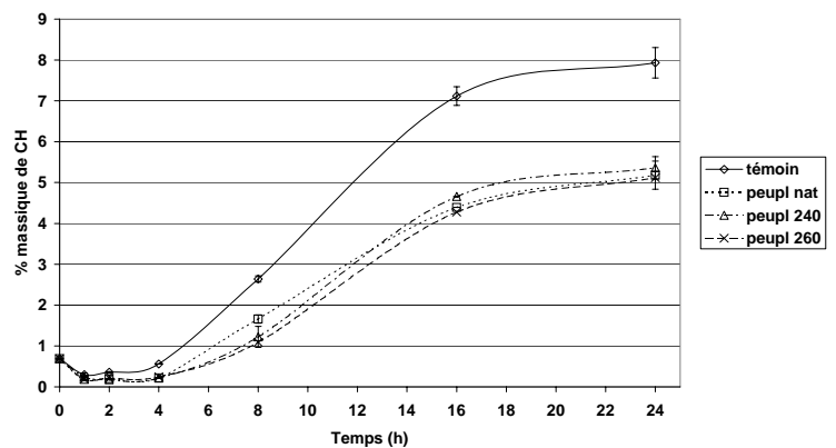
fig 2: évolution de la portlandite au cours du temps
