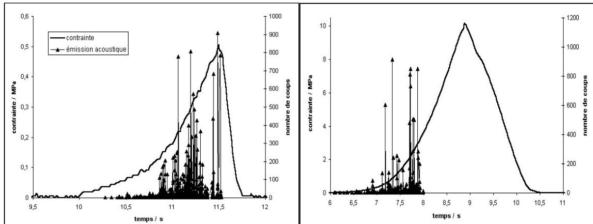
Fig. 4 Courbes contrainte et émission acoustique en fonction du temps pour le sable 2 – effet de la pression.
